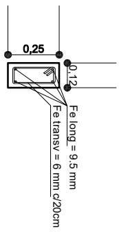
DETALLE DE VIGA CADENA
