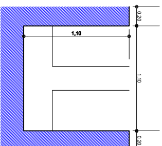
EXCAVACION ZAPATAS ESC: 1:50
