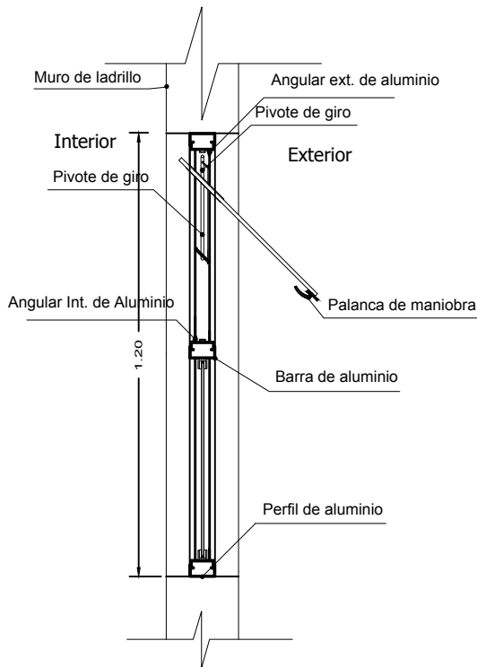
SECCION A-A
