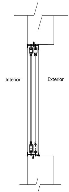
SECCION A-A
