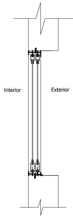
SECCION A-A
