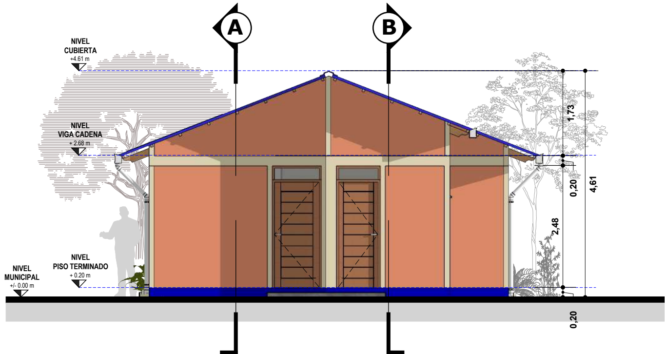
POSTERIOR ESC. 1:75
