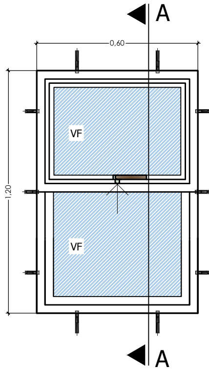
ELEVACION
