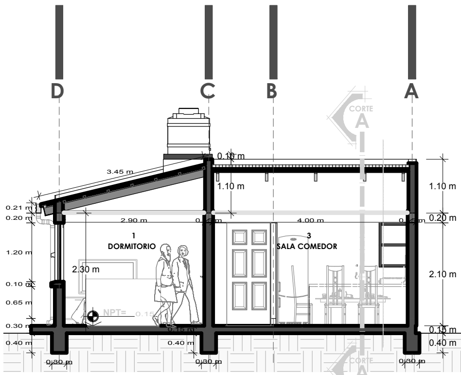
CORTE B-B
