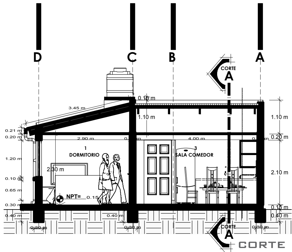
CORTE A-A
