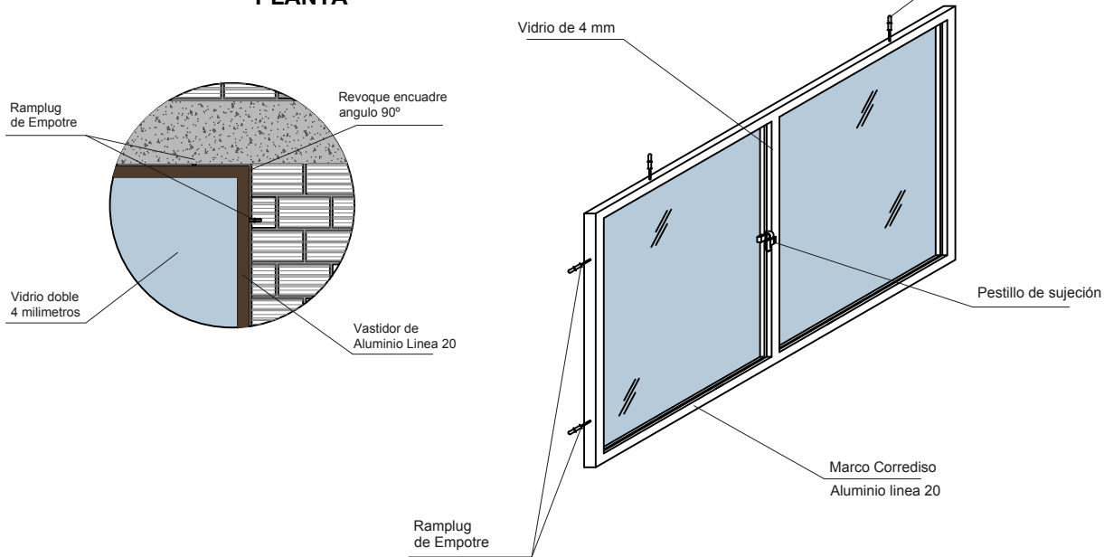
PLANTA
