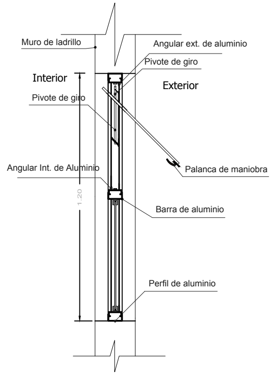
SECCION A-A
