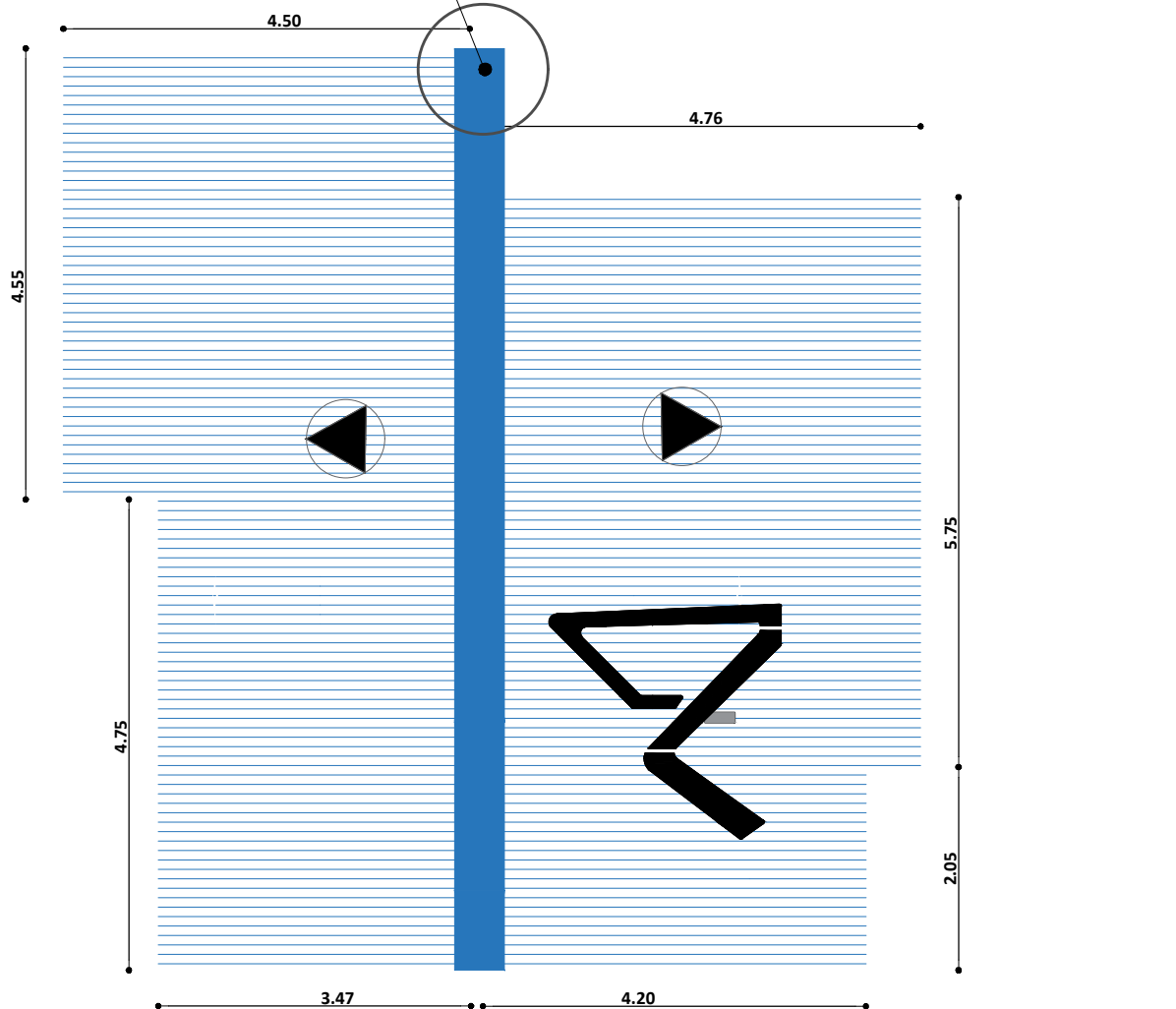
PLANO DE CUBIERTA ESC. 1:75
