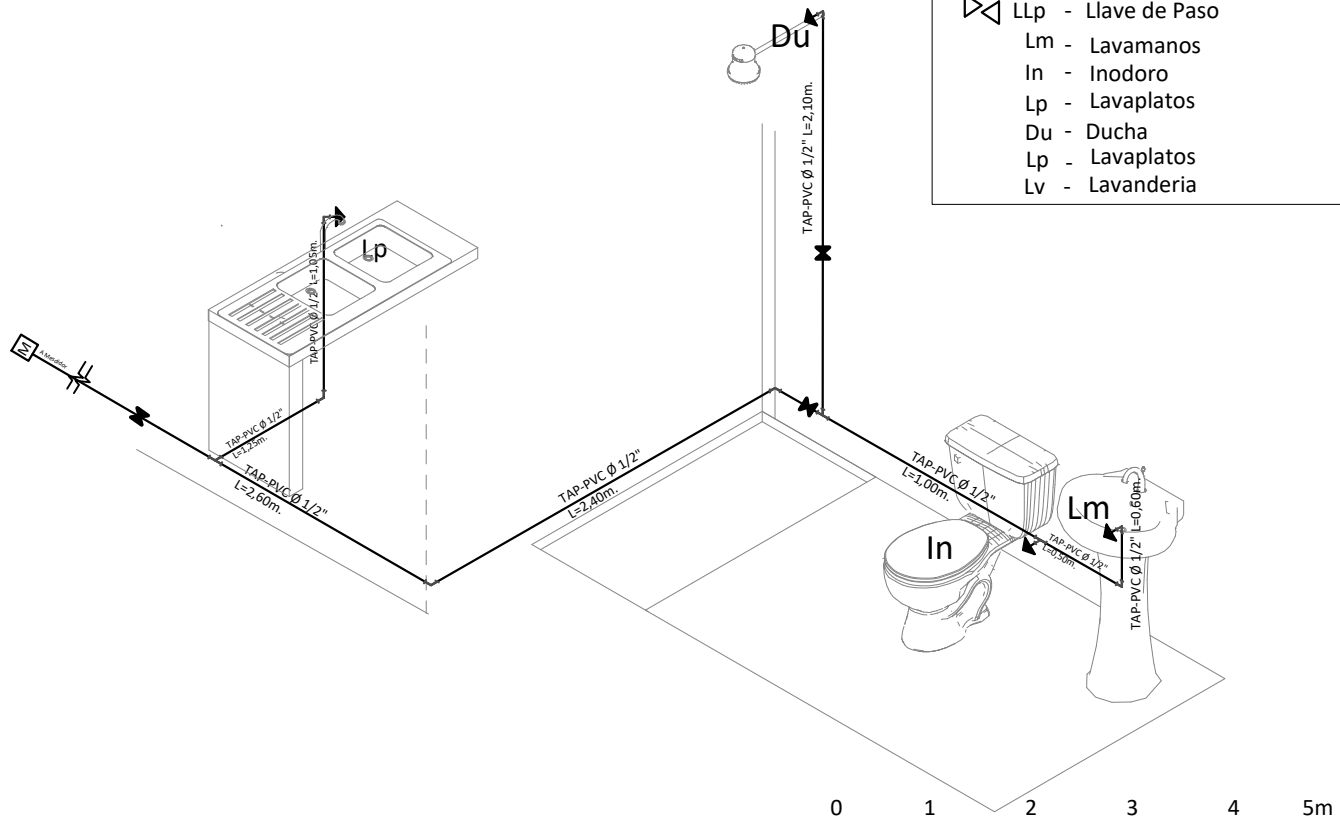
PLANO DE INSTALACION AGUA POTABLE ESC. 1:75
