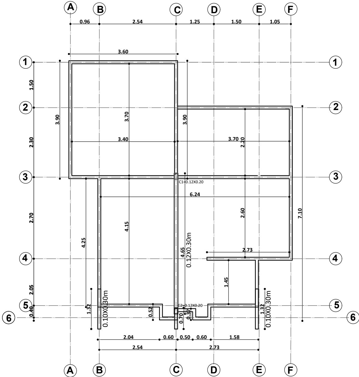
PLANO VIGA CADENA DE H°A°
