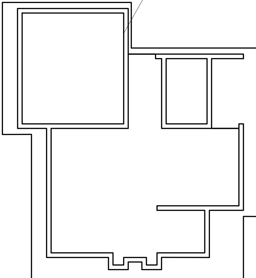
DETALLE DE ESQUINERO
