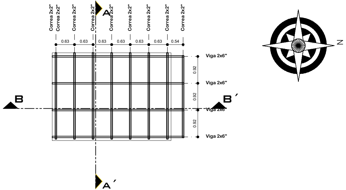
PLANO ESTRUCTURAL DE CUBIERTAS ESCALA: 1:75
