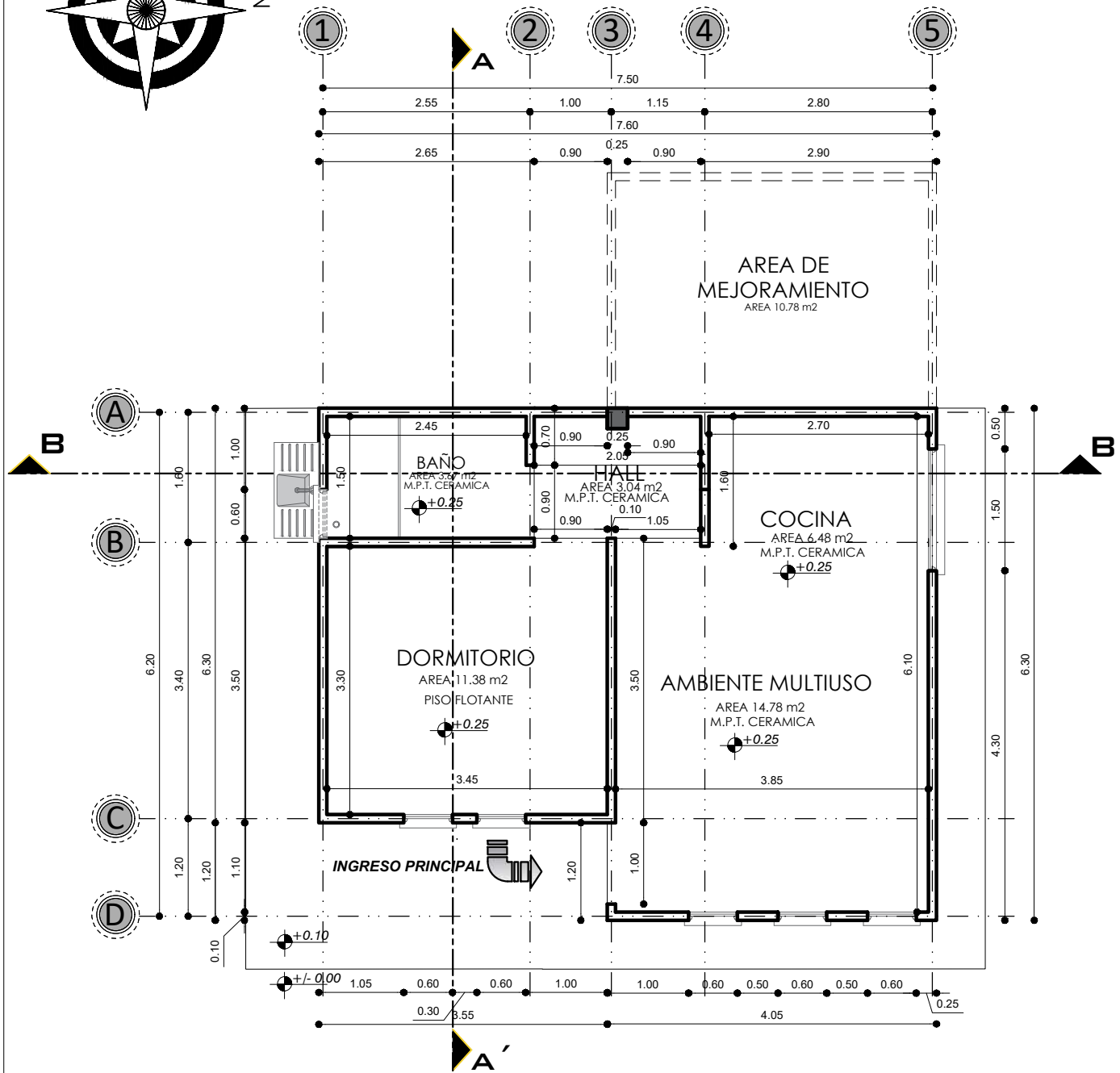
PLANTA ACOTADA ESCALA: 1:75
