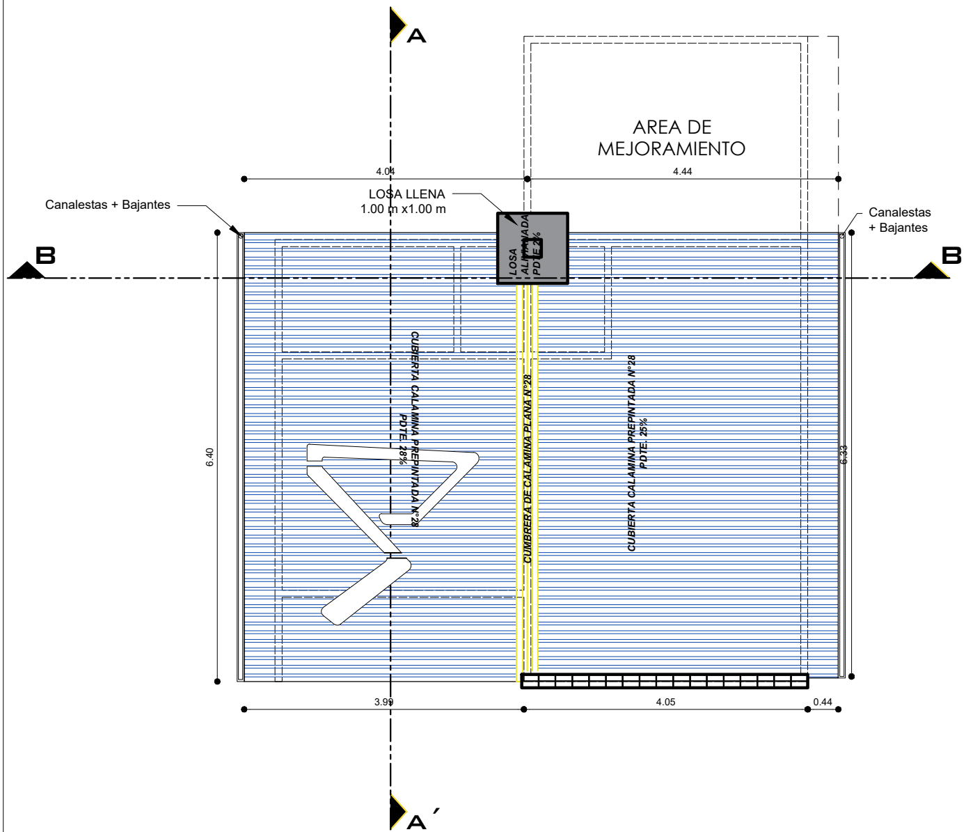
PLANO DE CUBIERTAS ESCALA: 1:75
