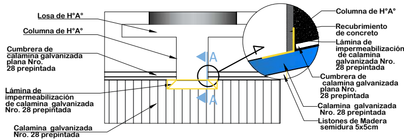
DETALLE DE IMPERMEABILIZACIÓN DE CUBIERTA ESC: 1:25
