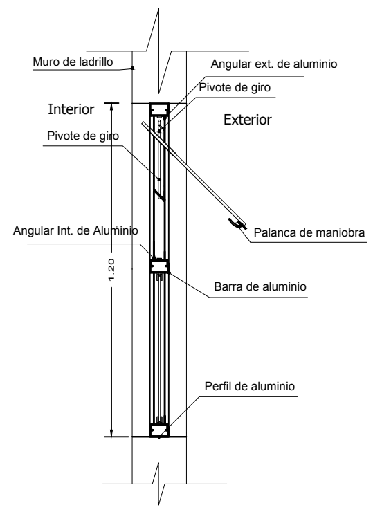
SECCION A-A
