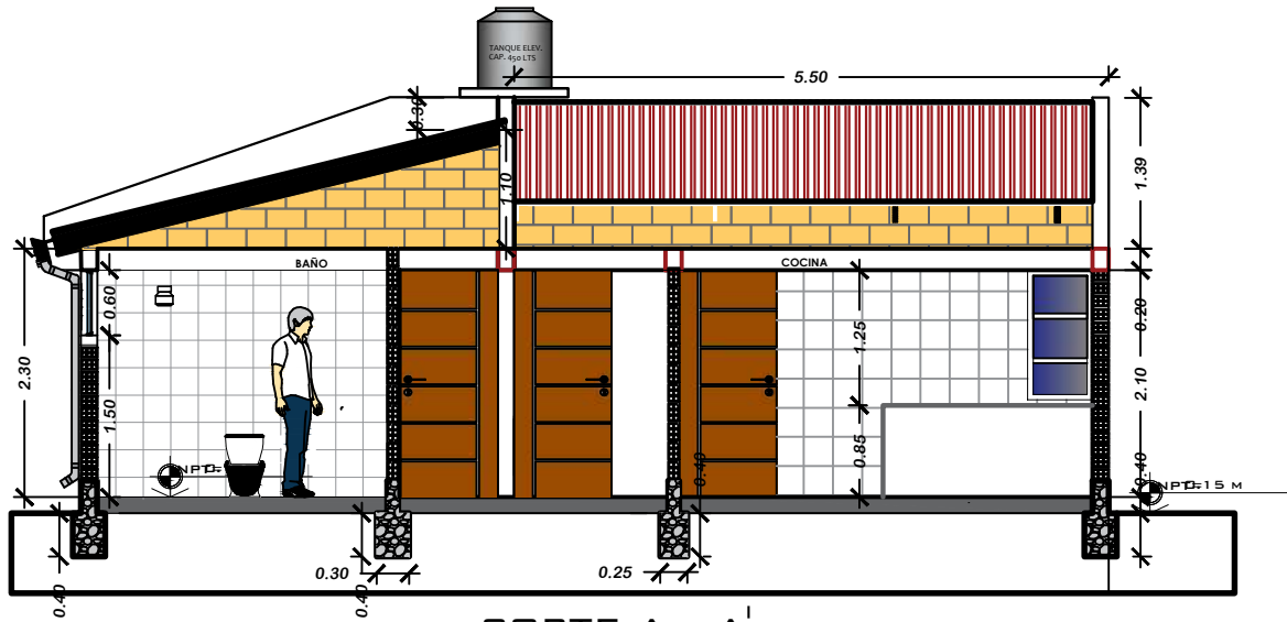
CORTE A - A I
