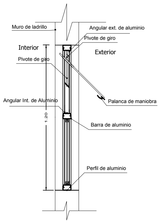
SECCION A-A
