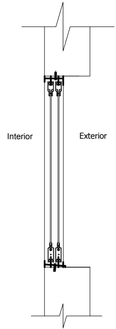
SECCION A-A
