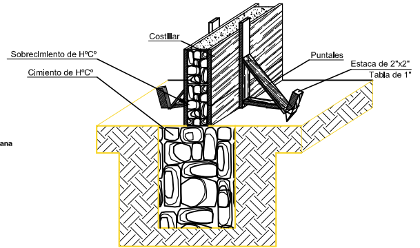
DETALLE ARMADO DE CIMIENTO Y SOBRECIMIENTO DE H° C°
