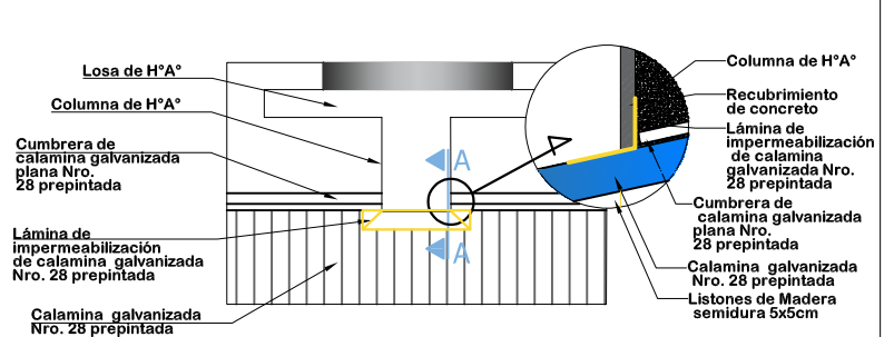
DETALLE DE IMPERMEABILIZACIÓN DE CUBIERTA ESC: 1:25
