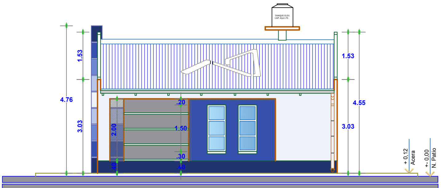
ELEVACION LATERAL
