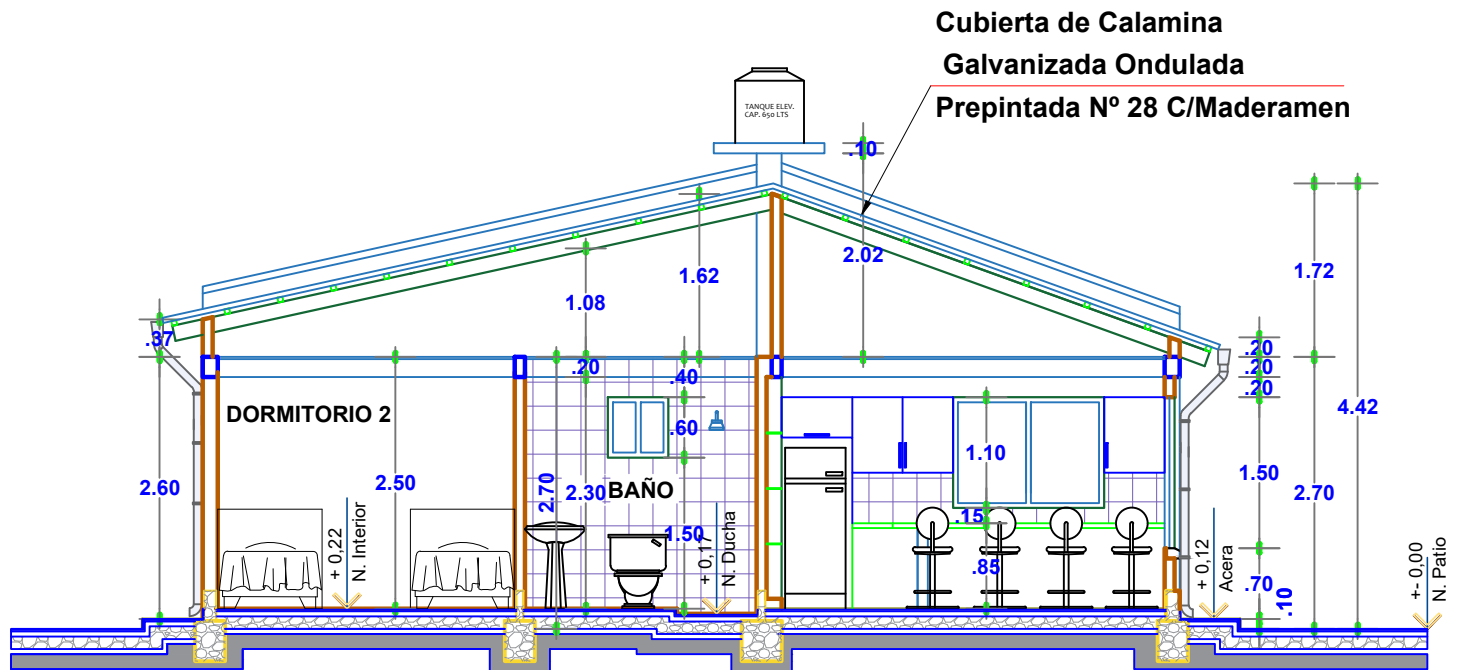
CORTE A-A'
