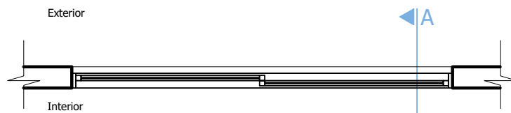
PLANTA
