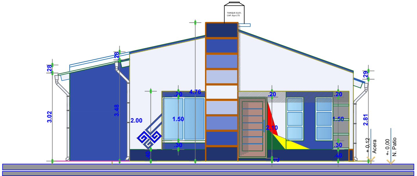
ELEVACION PRINCIPAL
