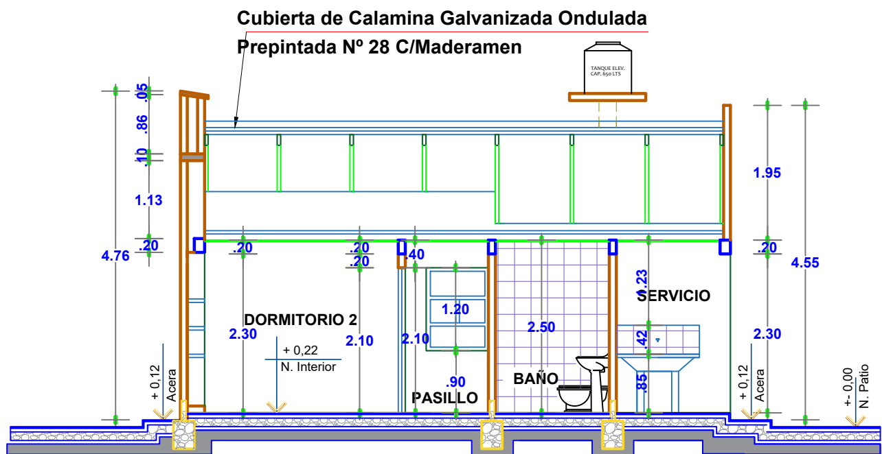
CORTE B-B'
