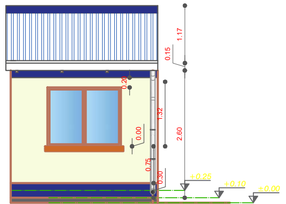
ELEVACION LATERAL ESCALA: 1:75
