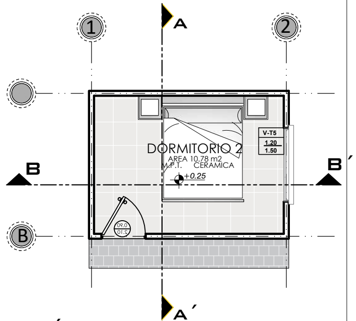
PLANTA AMOBLADA ESCALA: 1:75
