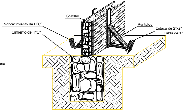
DETALLE ARMADO DE CIMIENTO Y SOBRECIMIENTO DE H² Cº
