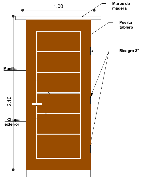
PUERTA 1,00x2,10
