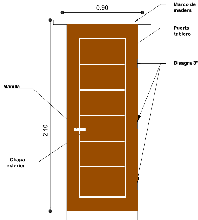
PUERTA 0,90x2,10
