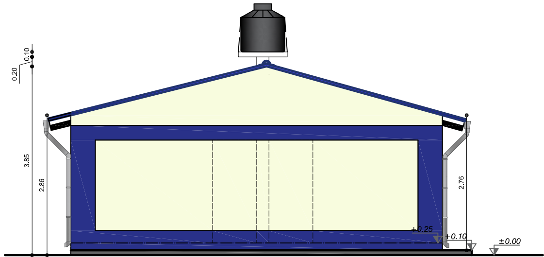
ELEVACION POSTERIOR ESCALA: 1:75
