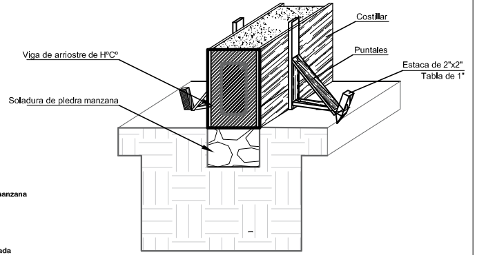
DETALLE ARMADO DE VIGA DE ARRIOSTRE H° A°
