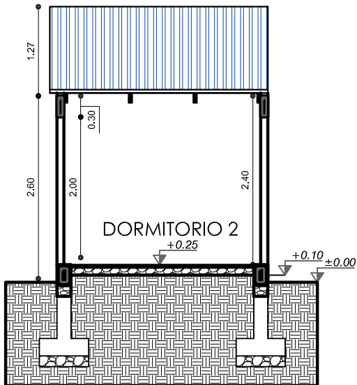
SECCION A-A I ESCALA: 1:75
