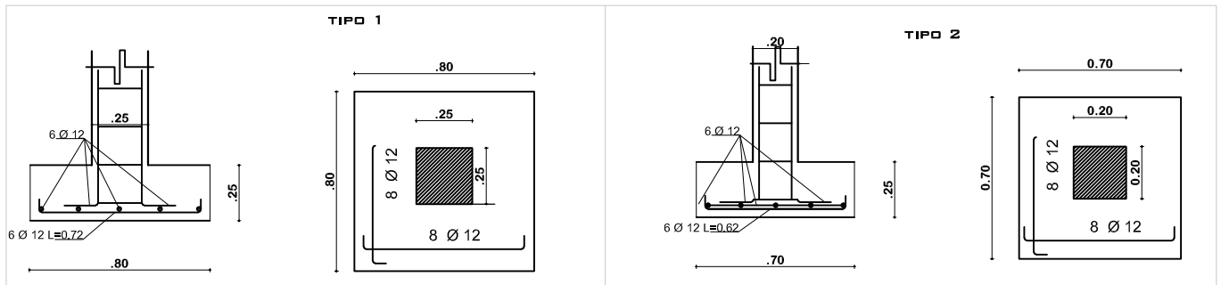
DETALLE DE LA ARMADURA EN ZAPATAS ESCALA: 1:30
