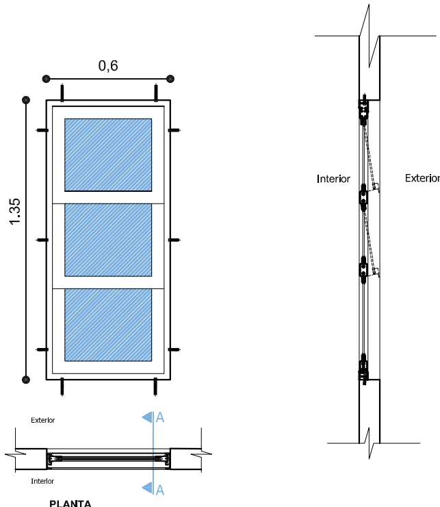
DETALLE VENTANA DE ALUMINIO 1,35 x 0,60
