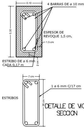
DETALLE DE VIGA 1
