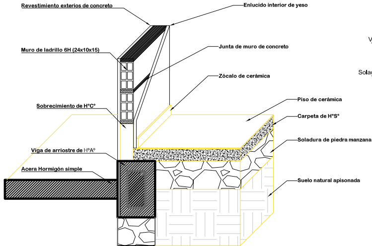
DETALLE SOBRECIMIENTO Y SUELO DE CERÁMICA
