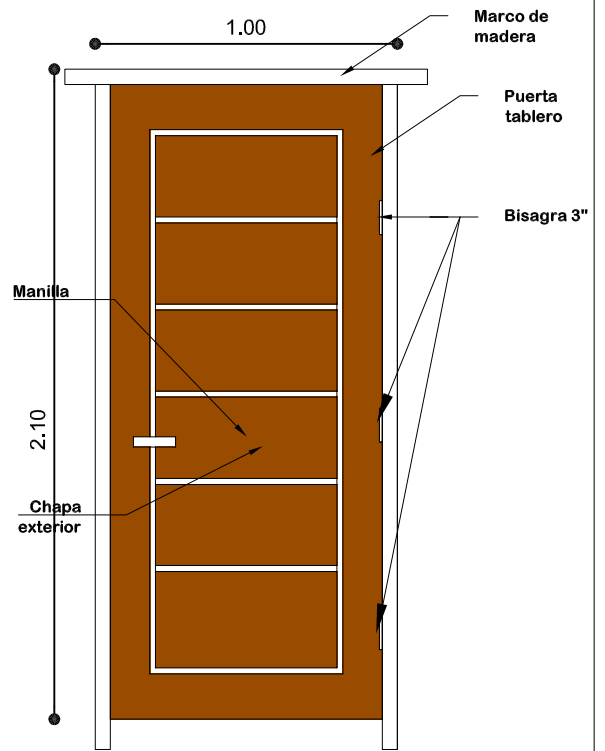
PUERTA 1,00x2,10
