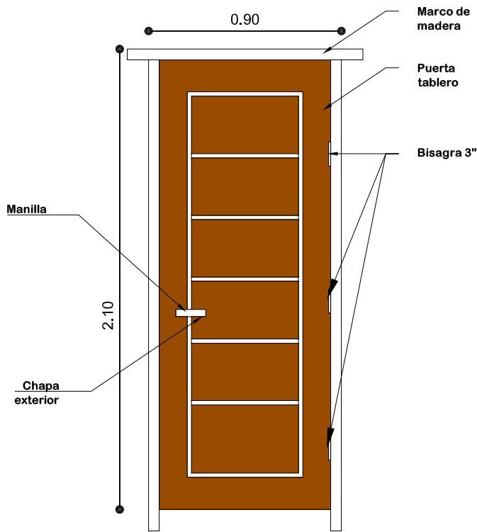
PUERTA 0,90x2,10
