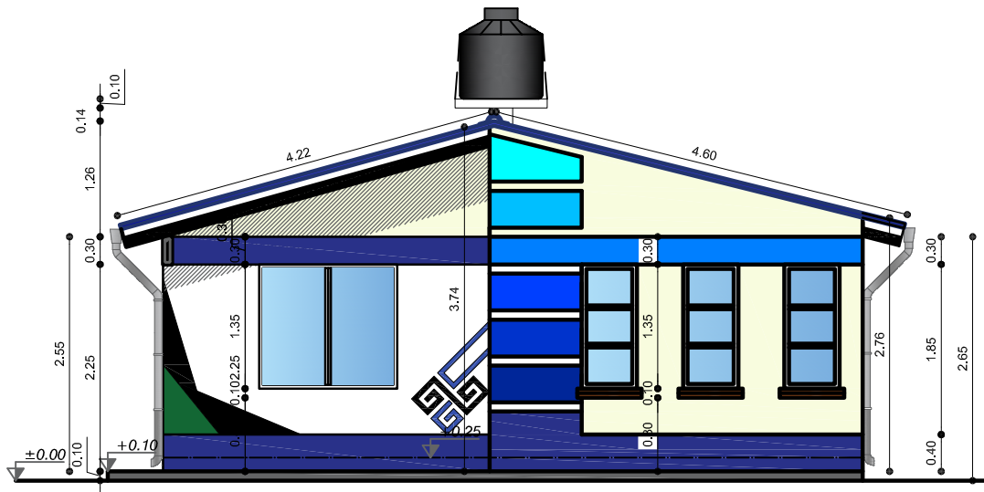
ELEVACION FRONTAL ESCALA: 1:75
