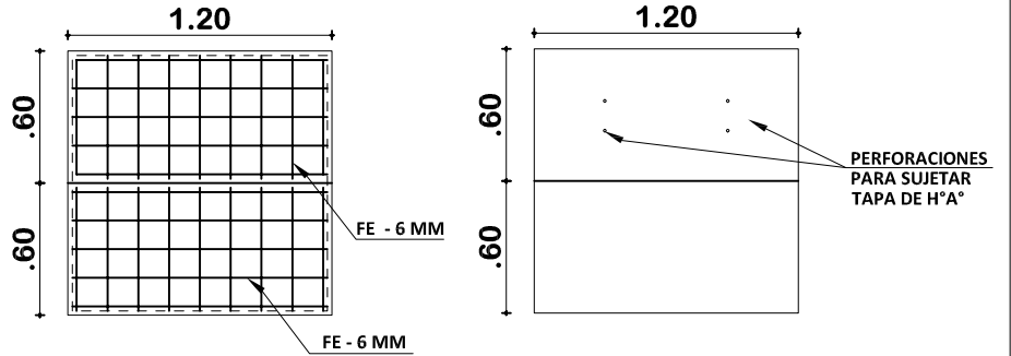
PLANTA
