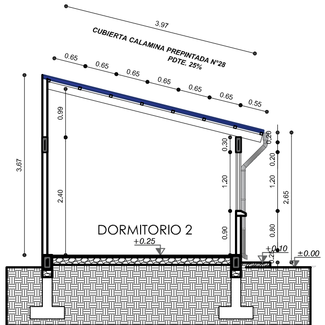
SECCION B-B I ESCALA: 1:75
