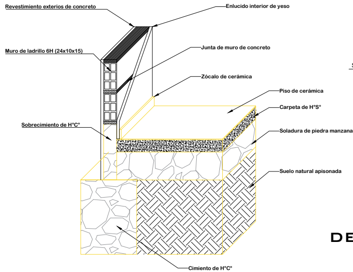
DETALLE CIMENTO Y SUELO DE CERÁMICA
