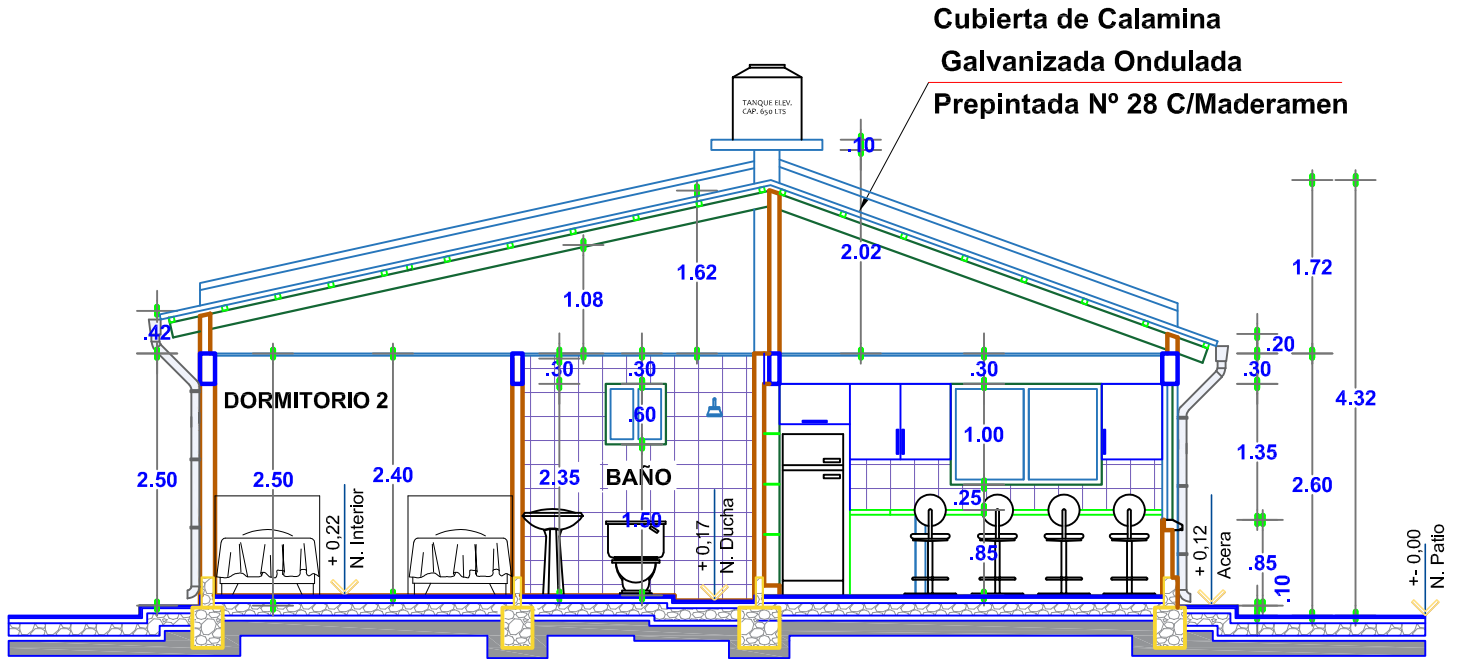
CORTE A-A'
