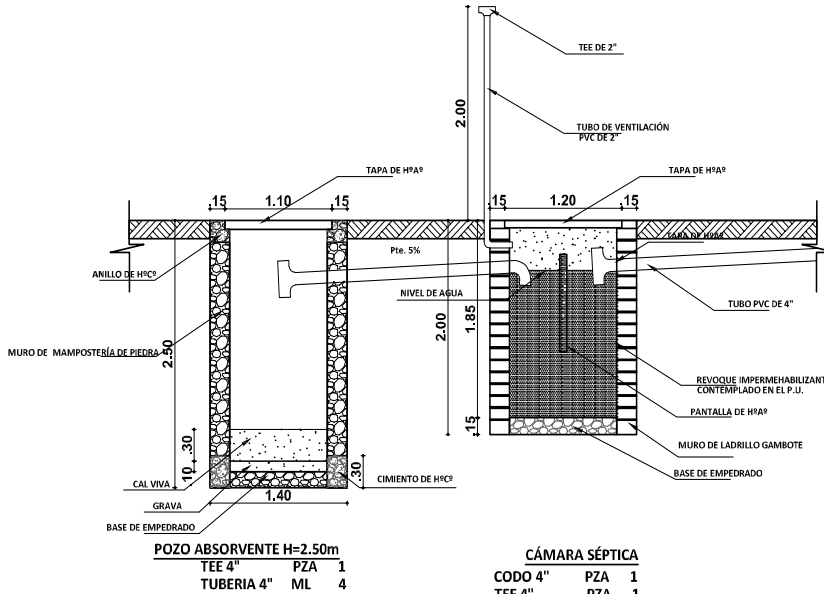
PLANO INSTALACION CAMARA Y POZO ABSORVENTE ESCALA: 1:75
