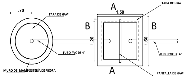
DETALLE CONSTRUCTIVOS POZO DE ABSORCION Y CAMARA SEPTICA ESCALA: 1:50
