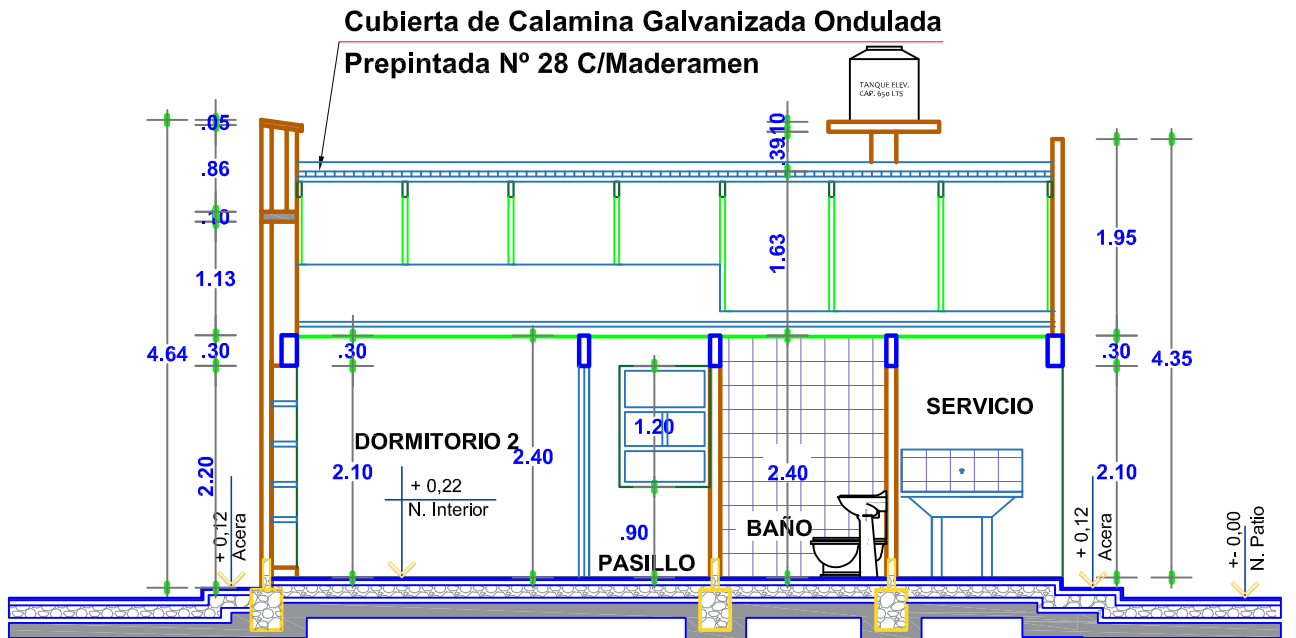
CORTE B-B'
