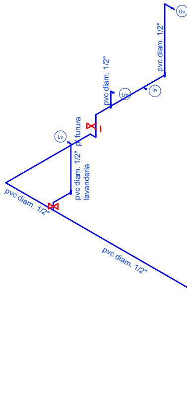
40 PLANO ESQUEMATICO ISOMETRICO - DE INSTALACION HIDRAULICA Scale: 1:100
