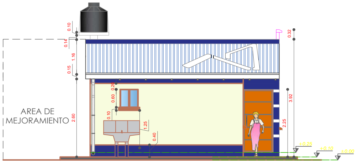
ELEVACION LATERAL IZQUIERDO
