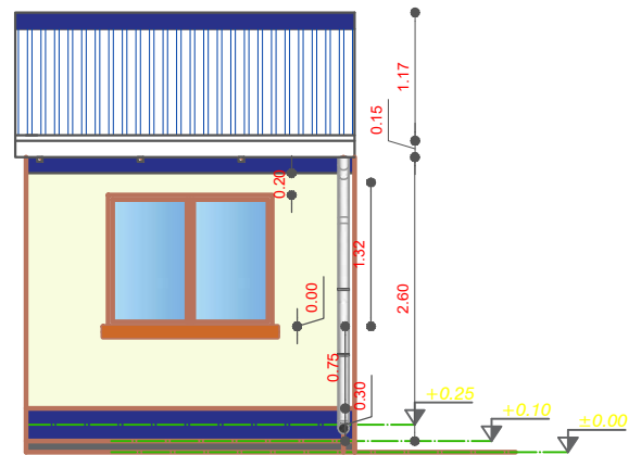
ELEVACION LATERAL ESCALA: 1:75
