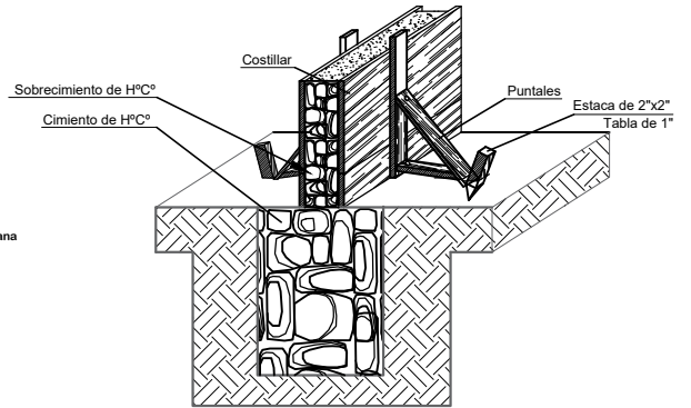
DETALLE ARMADO DE CIMIENTO Y SOBRECIMIENTO DE H² C²
