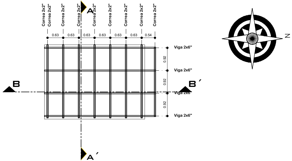
PLANO ESTRUCTURAL DE CUBIERTAS ESCALA: 1:75
