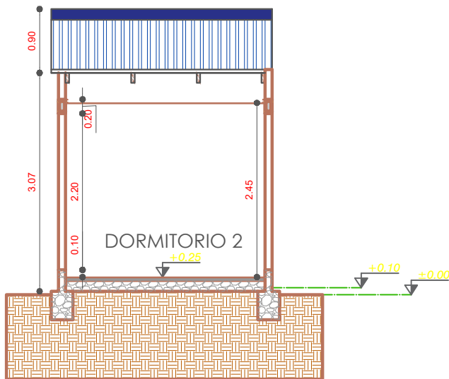
SECCION A-A' ESCALA: 1:75
