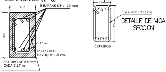
DETALLE VIGA 2 EJE 3 TRAMO A-B
