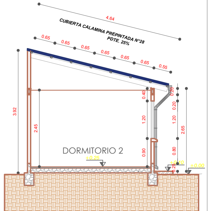
SECCION B-B' ESCALA: 1:75
