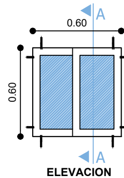
ELEVACION
