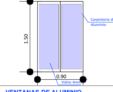
VENTANAS DE ALUMINIO LINEA 20 CON VIDRIO 4 mm
