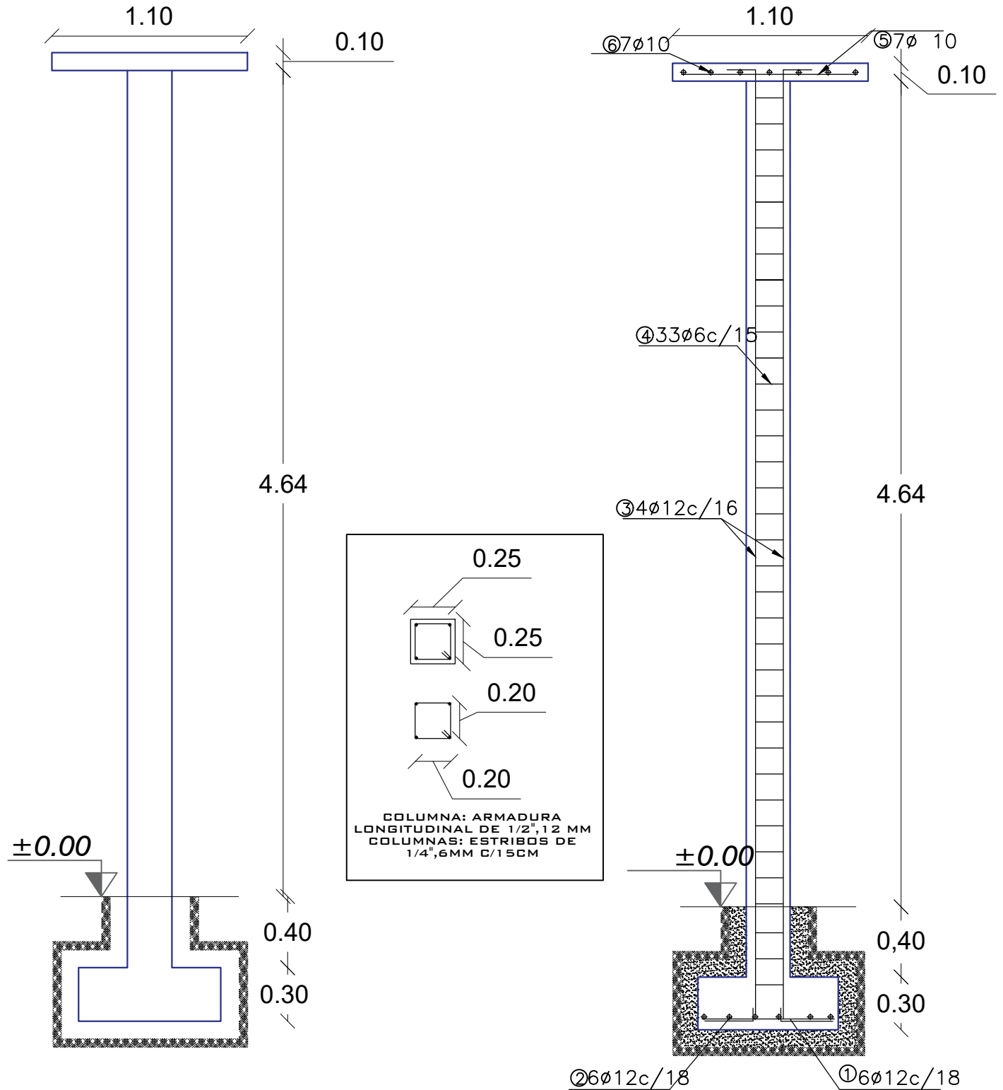
DETALLE ARMADURA DE COLUMNA ESC: 1:30
