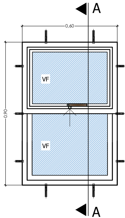
ELEVACION
