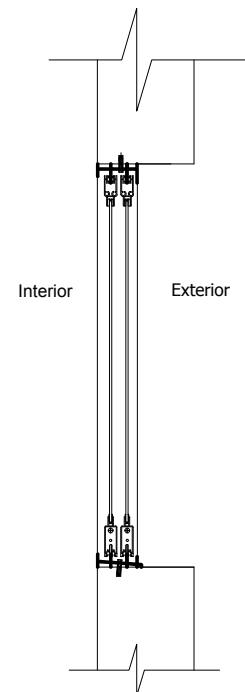
SECCION A-A
