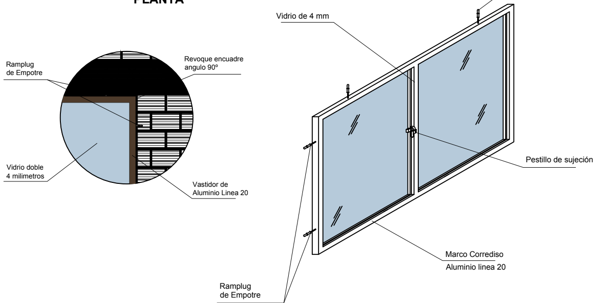
PLANTA
