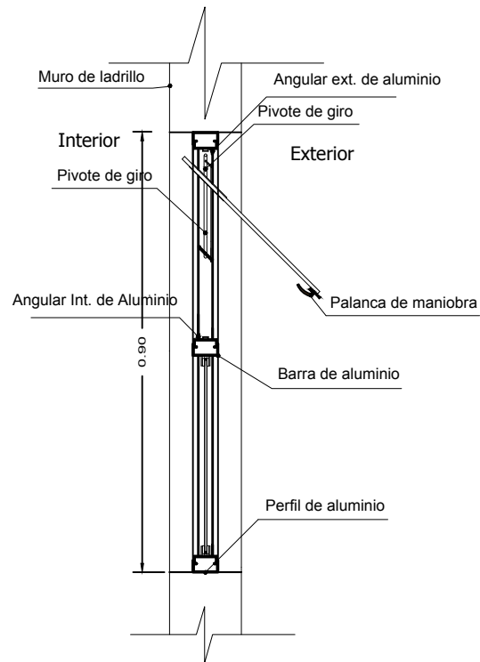
SECCION A-A
