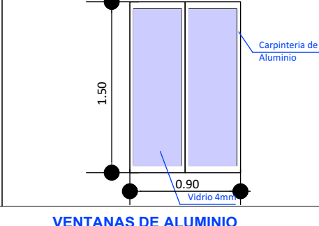
VENTANAS DE ALUMINIO LINEA 20 CON VIDRIO 4 mm
