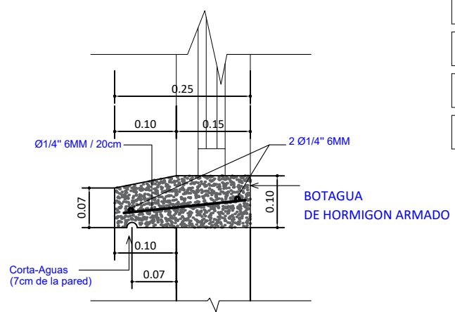
DETALLE DE BOTAGUA ESC. 1:20
