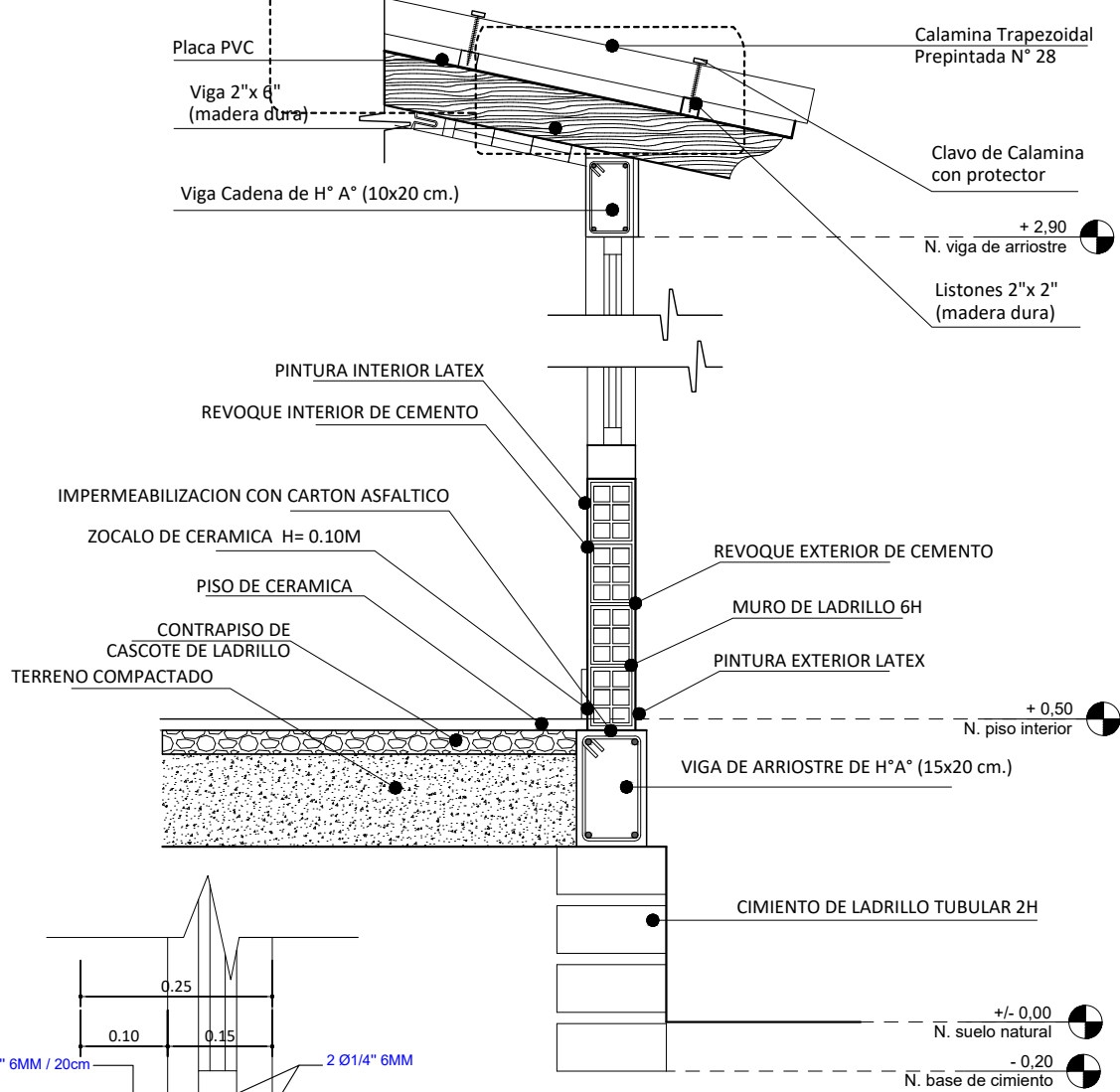
CORTE DE BORDE ESC. 1:20
