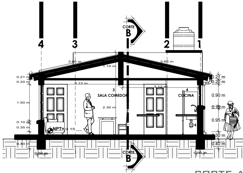
CORTE A-A
