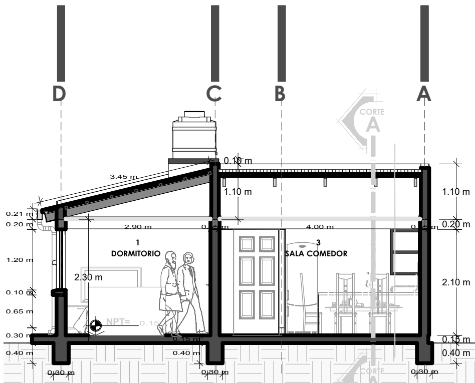
CORTE B-B
