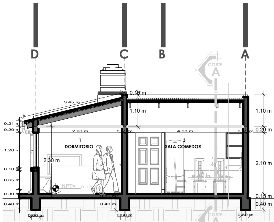
CORTE B-B
