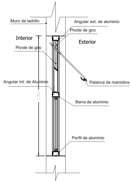
SECCION A-A
