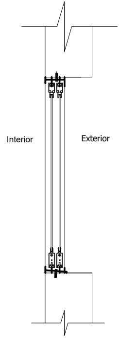
SECCION A-A
