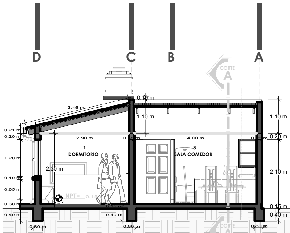
CORTE B-B
