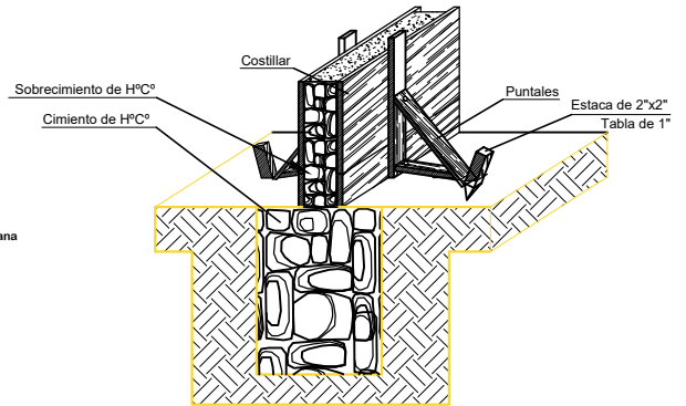
DETALLE ARMADO DE CIMIENTO Y SOBRECIMIENTO DE H 3 C 3
