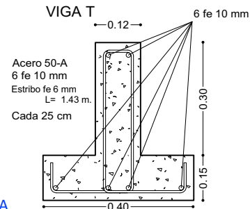
SECCION VIGA T
