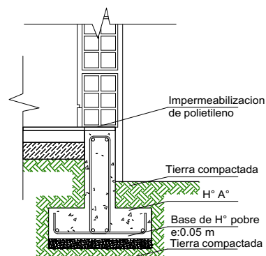
SECCIÓN ESTRIBO
