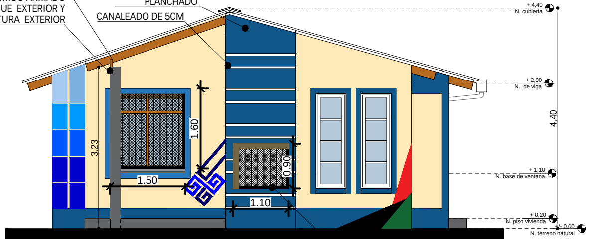
ELEVACION FRONTAL
