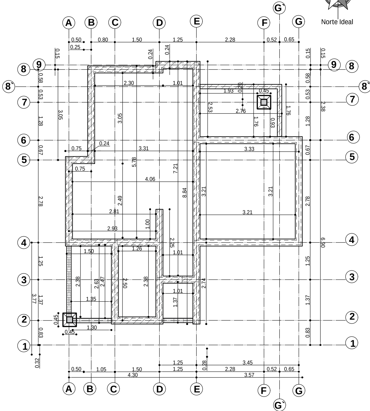
PLANO EXCAVACION-CIMIENTOS ESC. 1:75
