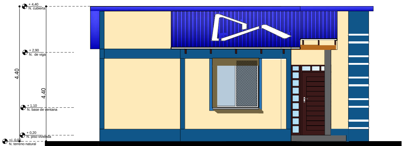
ELEVACION LATERAL DERECHA
