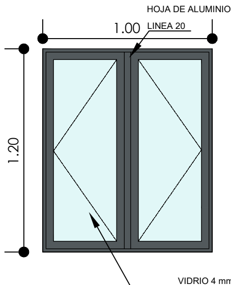
DETALLE DE VENTANA ESC. 1:25
