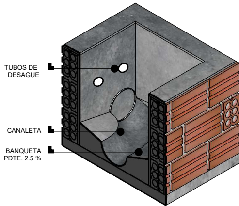
DETALLE CAMARA INSPECCION ESC. 1:25
