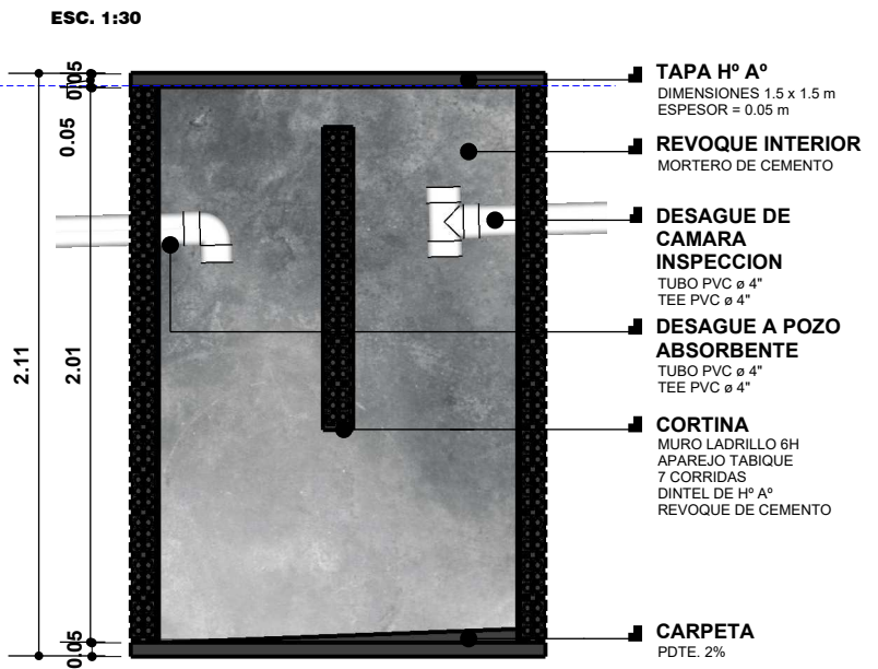
DETALLE CAMARA SEPTICA ESC. 1:30
