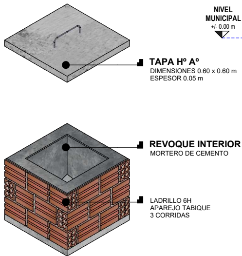
DETALLE CAMARA INSPECCION ESC. 1:25
