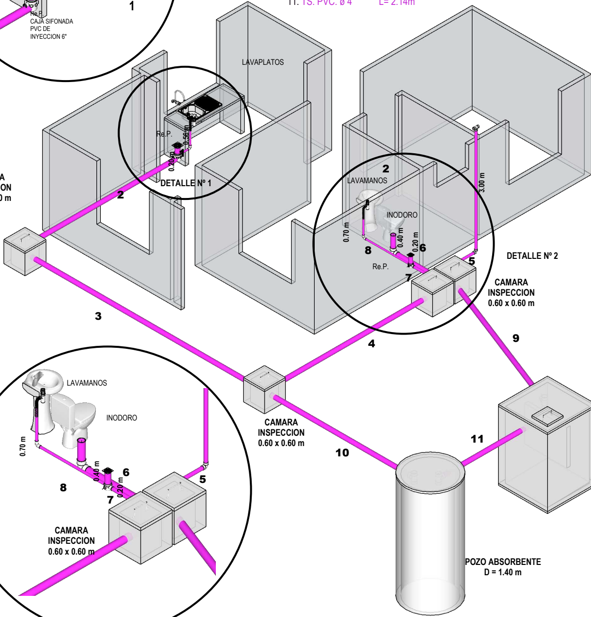
DETALLE N° 2
