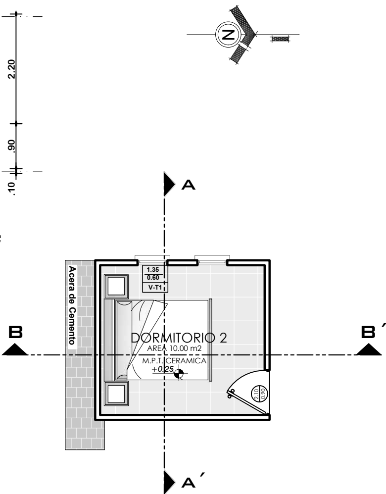
PLANTA AMOBLADA ESCALA: 1:75
