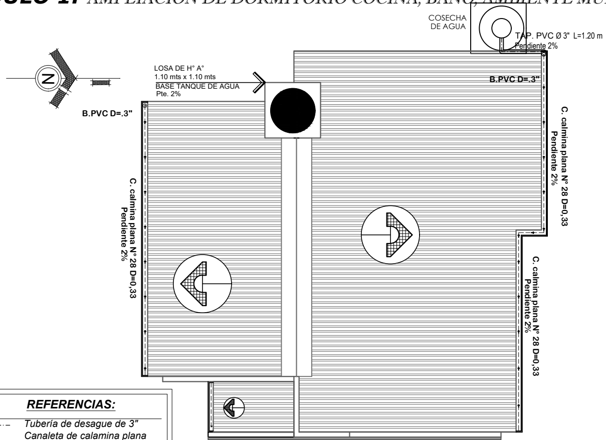
INSTALACION PLUVIAL ESCALA: 1:75
