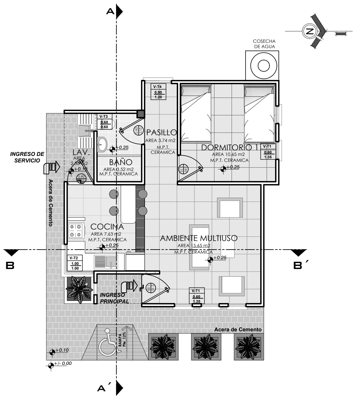
PLANTA AMOBLADA ESCALA: 1:75
