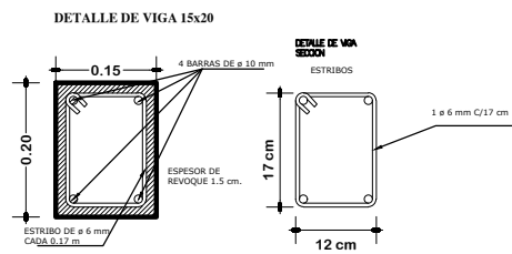
PLANTA DE VIGA DE H°A° ESCALA: 1:75
