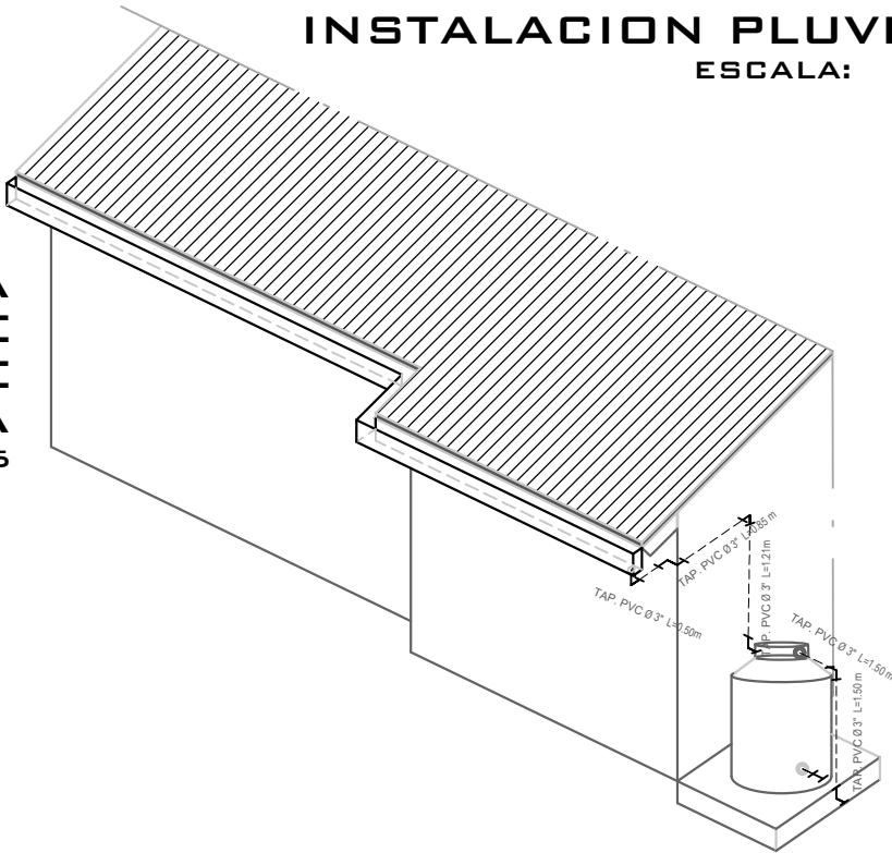
ISOMETRIA INSTALACION DE COSECHA DE AGUA ESCALA: 1:75
