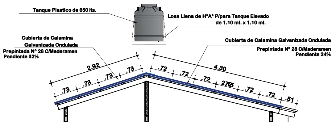
PLANO DE ESTRUCTURA MADERAMEN ESCALA: 1:75
