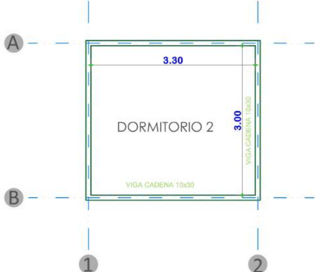
PLANO DE VIGA DE HºAº ESCALA: 1:75
