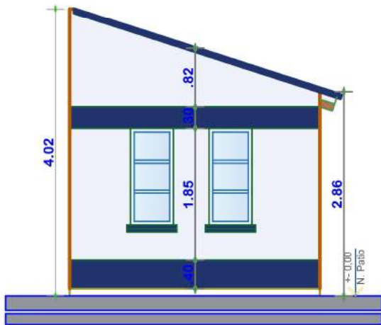
ELEVACION FRONTAL ESCALA: 1:75
