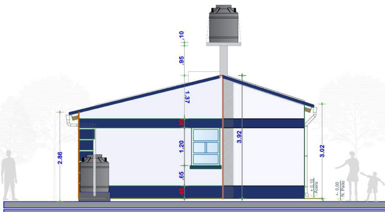
ELEVACION POSTERIOR ESCALA: 1:75
