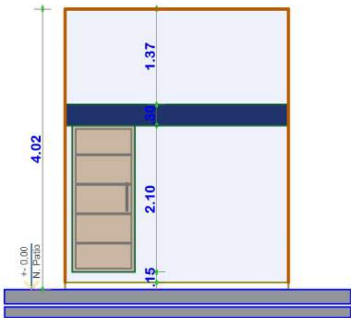
ELEVACION LATERAL ESCALA: 1:75
