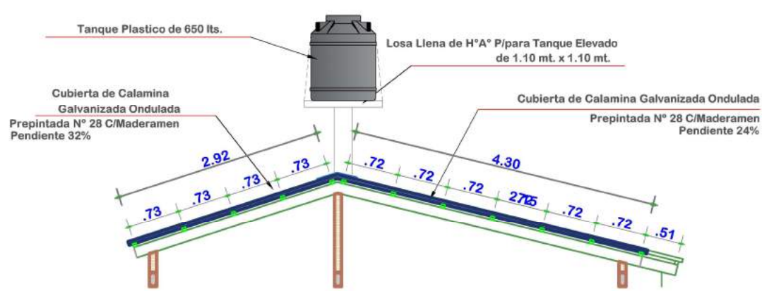
PLANO DE ESTRUCTURA MADERAMEN ESCALA: 1:75
