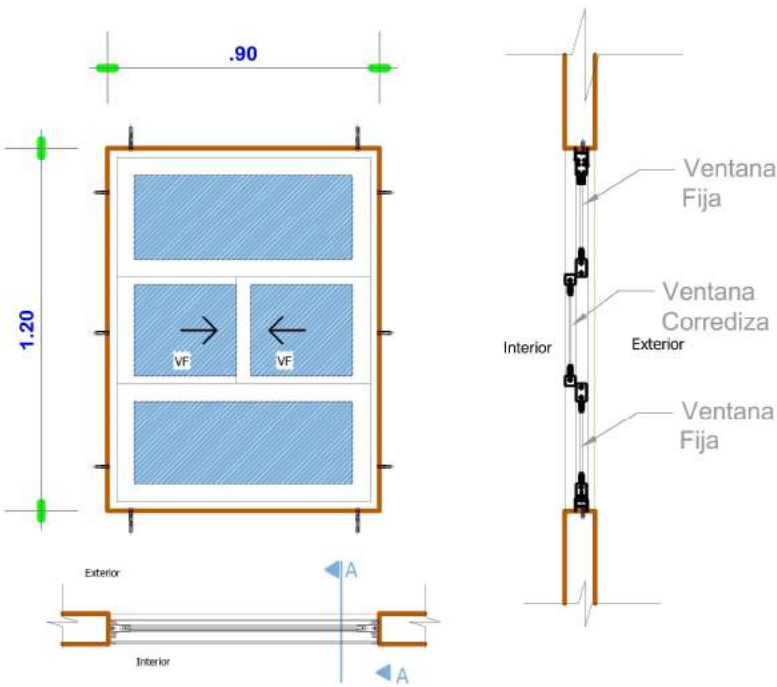
VENTANA TIPO 4 DETALLE VENTANA DE ALUMINIO 0.90 x 1.20 ESC: 1:25
