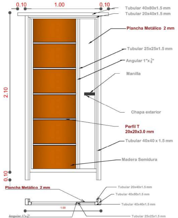
PUERTA 1.00 x 2,10
