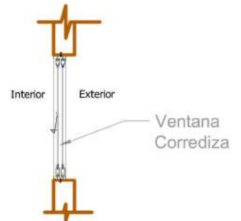
SECCION A-A
