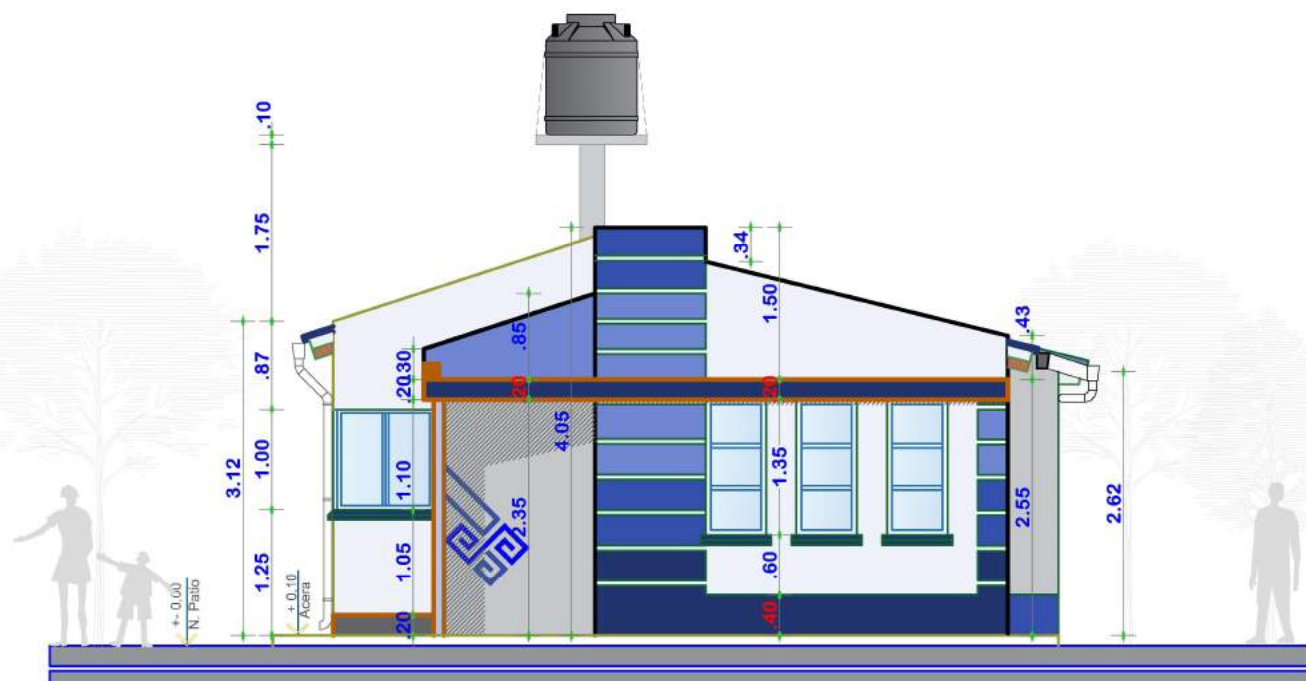
ELEVACION FRONTAL ESCALA: 1:75
