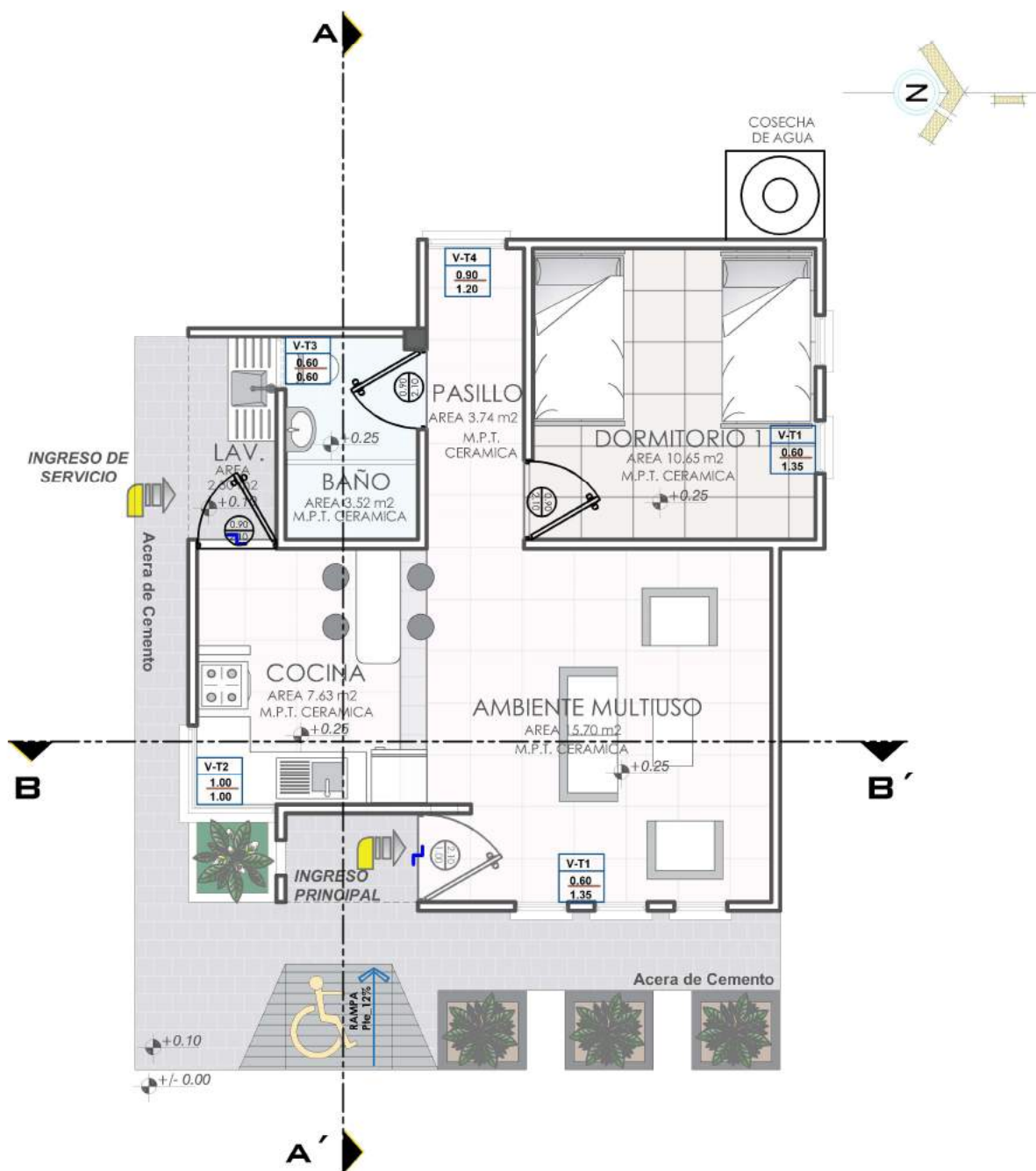
PLANTA AMOBLADA ESCALA: 1:75
