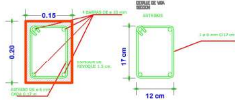
PLANTA DE VIGA DE H°A° ESCALA: 1:75
