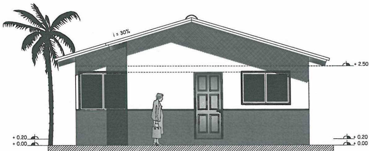
ELEVACIÓN POSTERIOR ESC. 1:75
