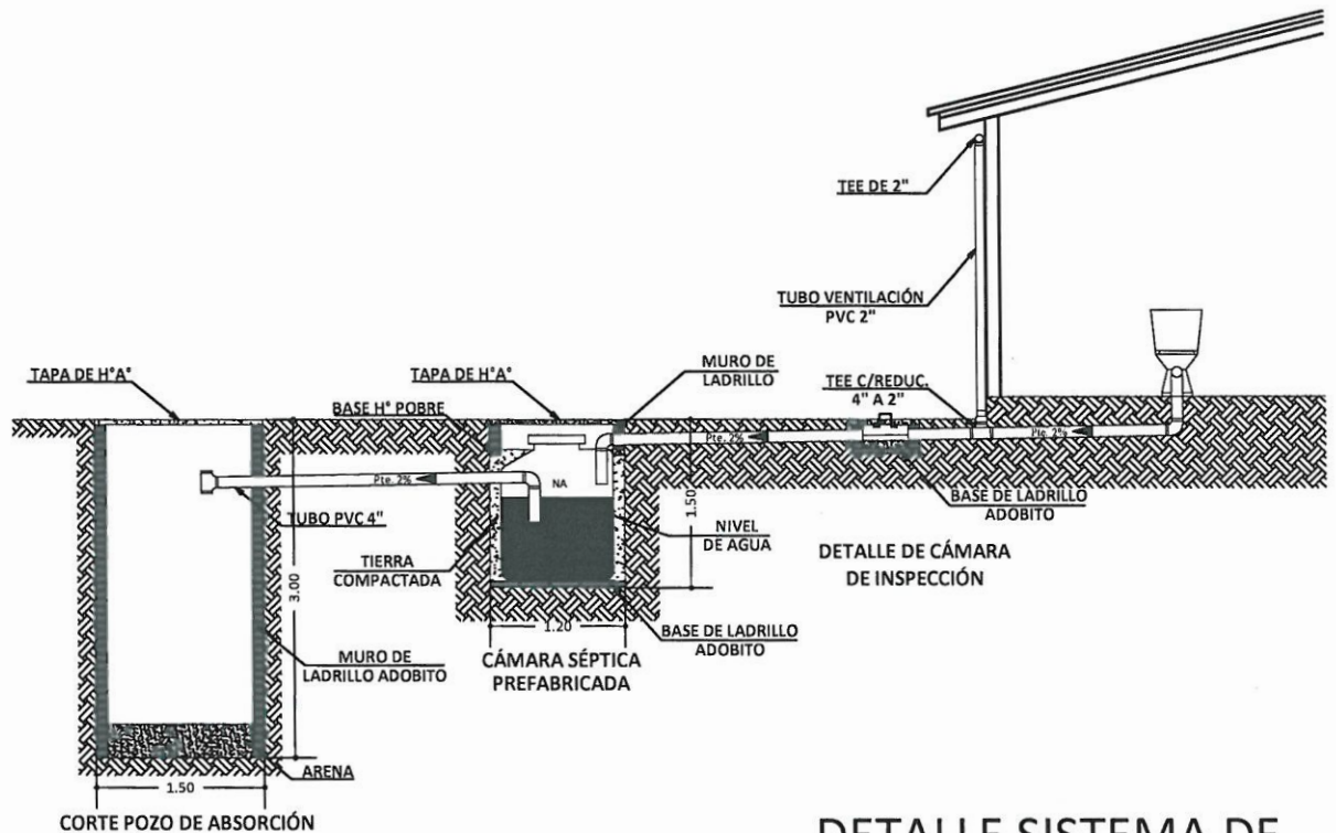
DETALLE SISTEMA DE DESCARGA - CORTE S/Esc.
