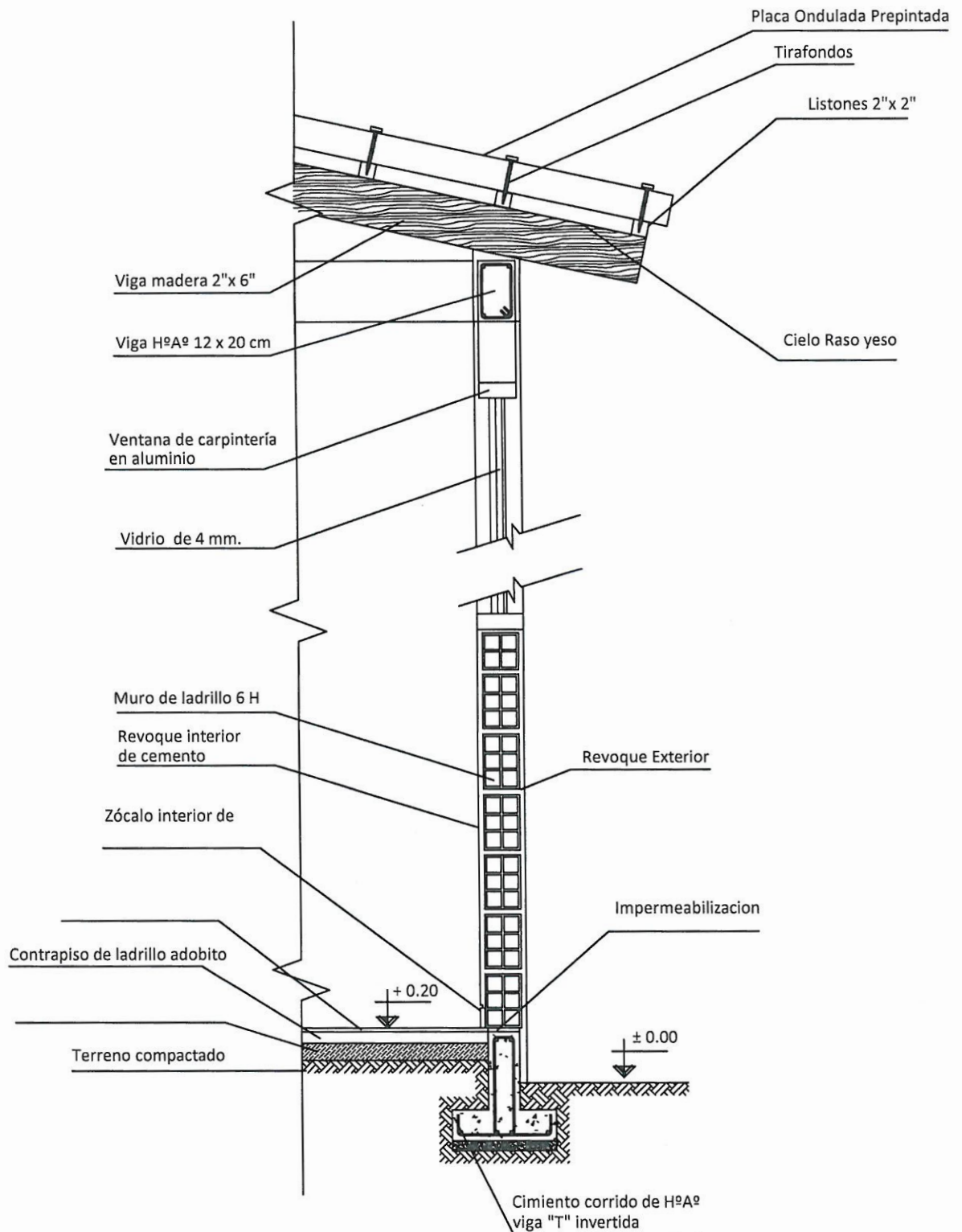
CORTE DE BORDE ESC. 1:20
