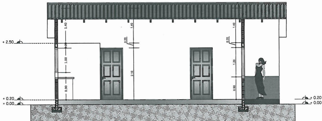
SECCIÓN A-A' ESC. 1:75
