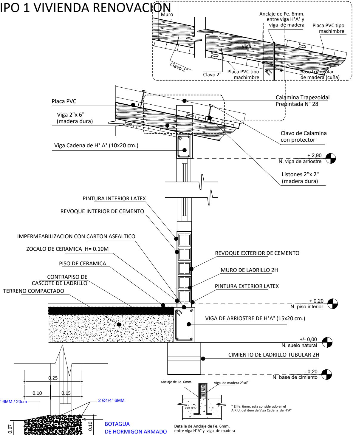
CORTE DE BORDE ESC. 1:20
