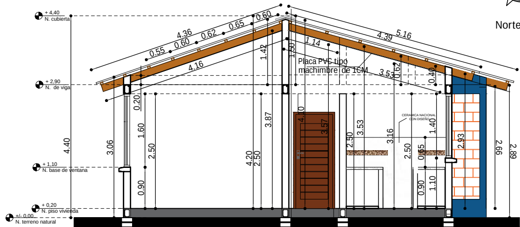
CORTE A - A' ESC. 1:75
