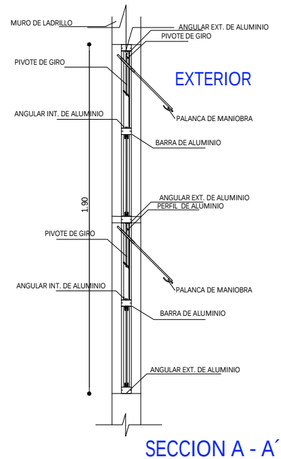
Ventana Tipo 4
