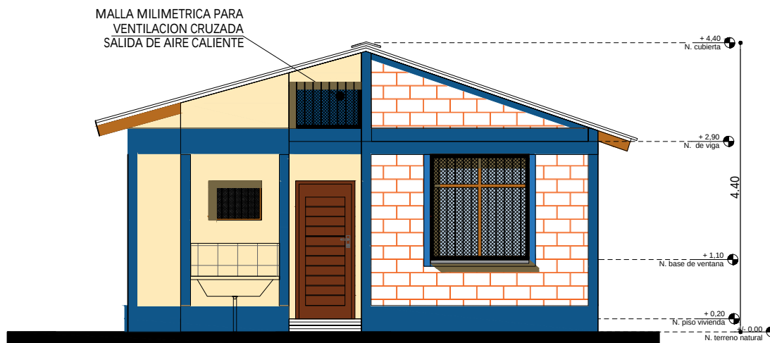
ELEVACION POSTERIOR SC. 1:75
