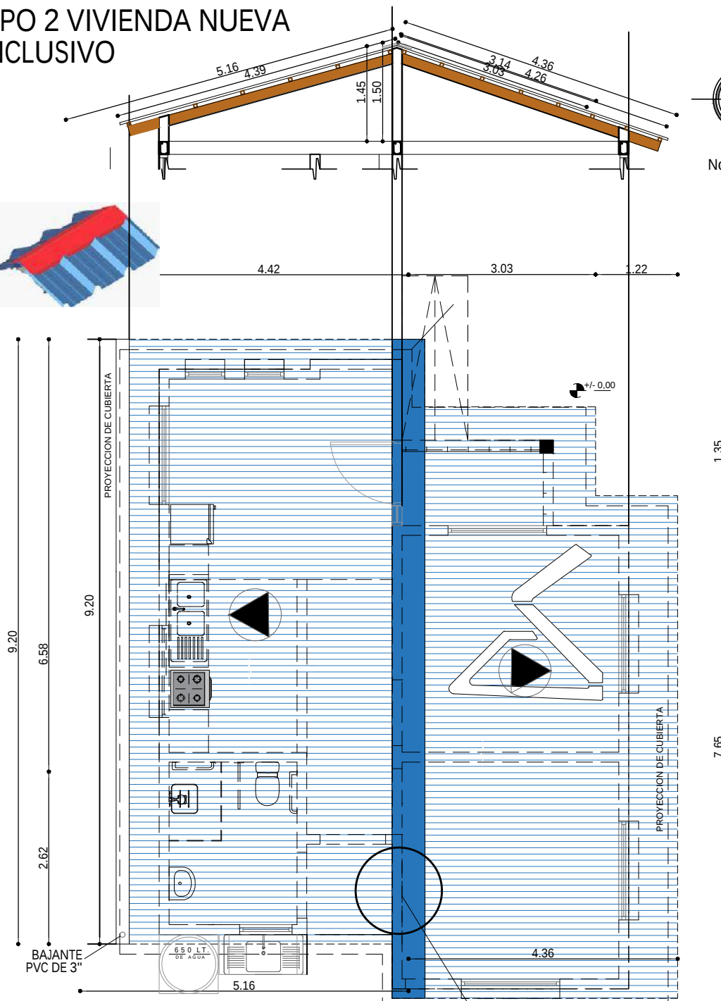
PLANO DE CUBIERTA ESC. 1:75
