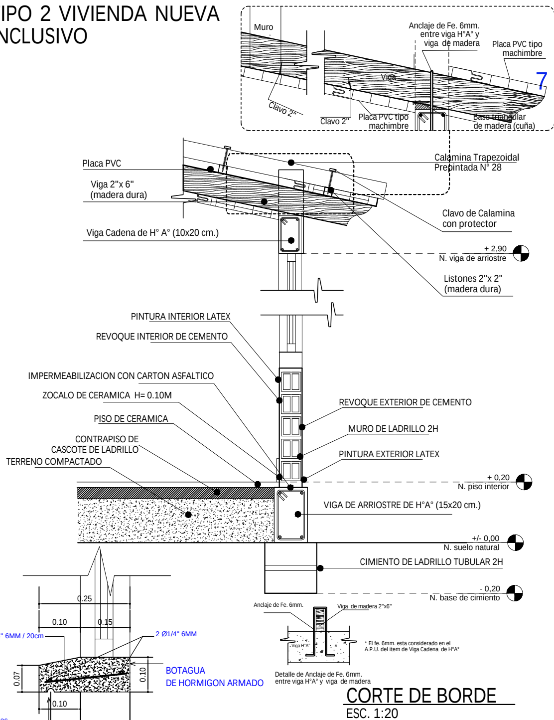
DETALLE DE BOTAGUA ESC. 1:20
