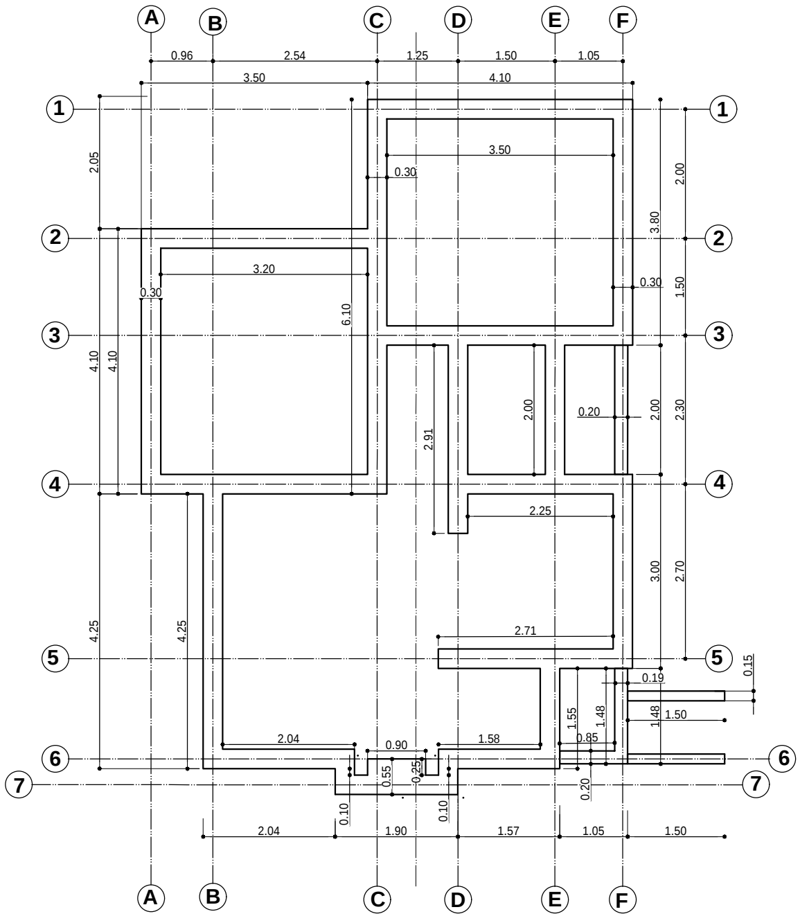
PLANO EXCAVACION-CIMENTOS ESC. 1:75
