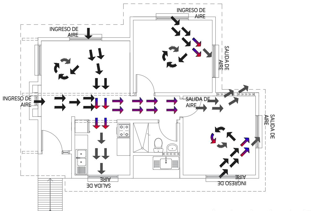
PLANTA CIRCULACION CRUZADA DE AIRE ESC. 1:100
