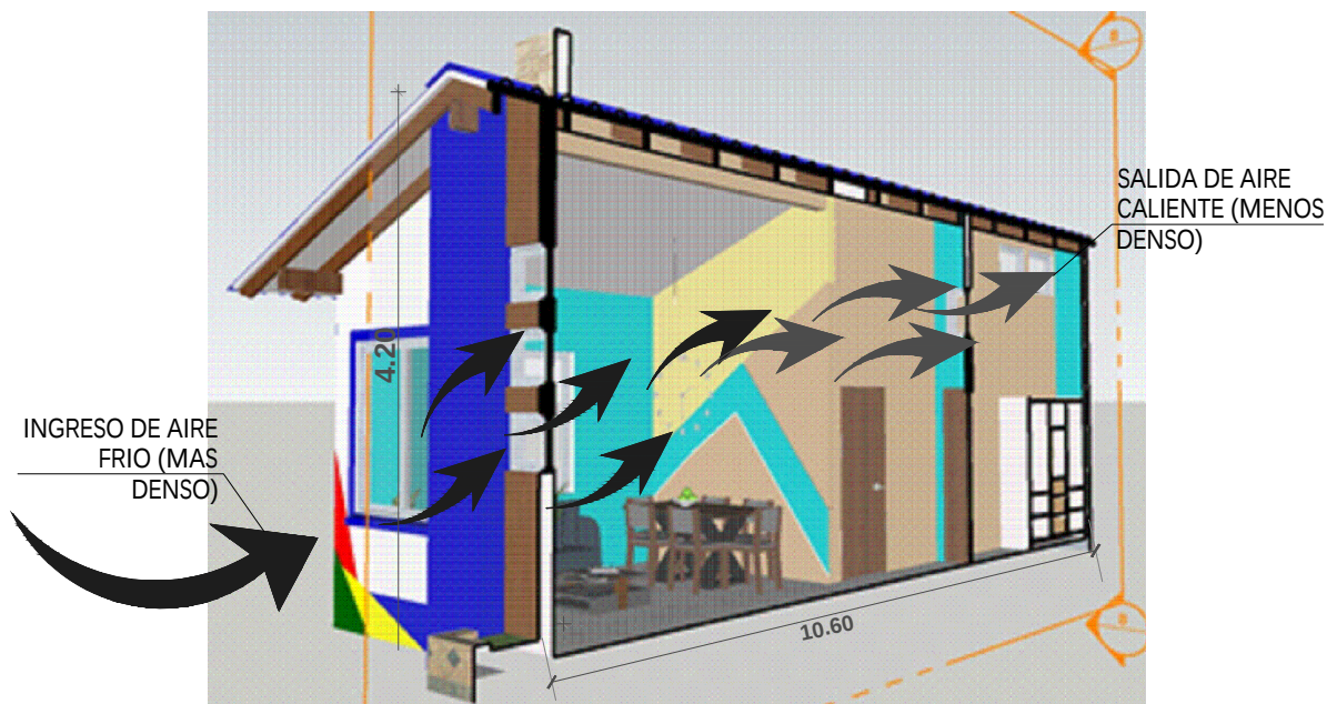
ESQUEMA PASILLO DE CIRCULACION GRUZADA ESC. S/E
