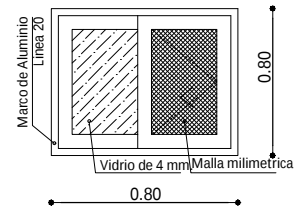
Ventana Tipo 3
