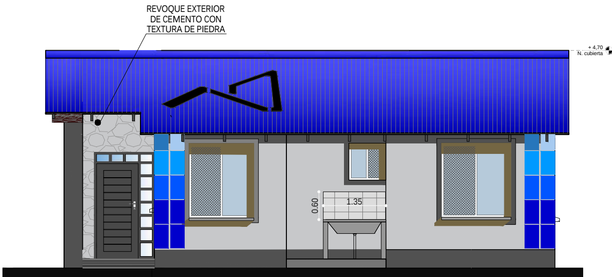
ELEVACION FRONTAL ESC. 1:75
