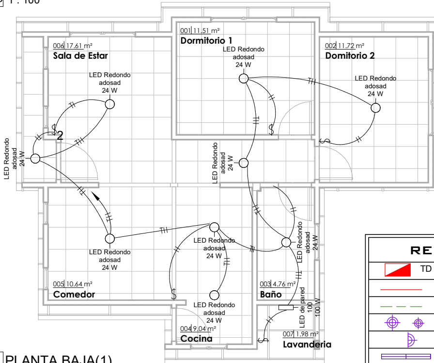
2 PLANTA BAJA(1) AR-15 1 : 100
