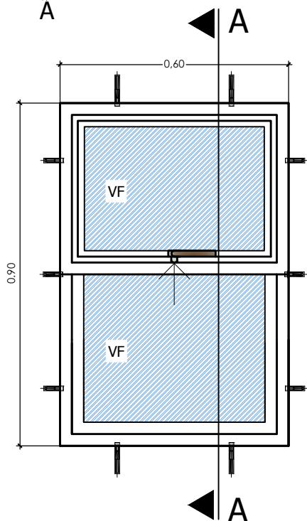
ELEVACION
