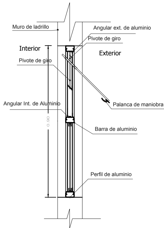
SECCION A-A
