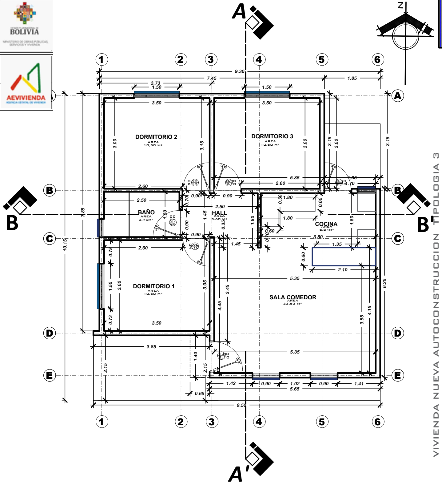
PLANTA ACOTADA
