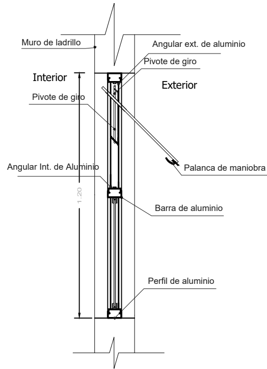
SECCION A-A
