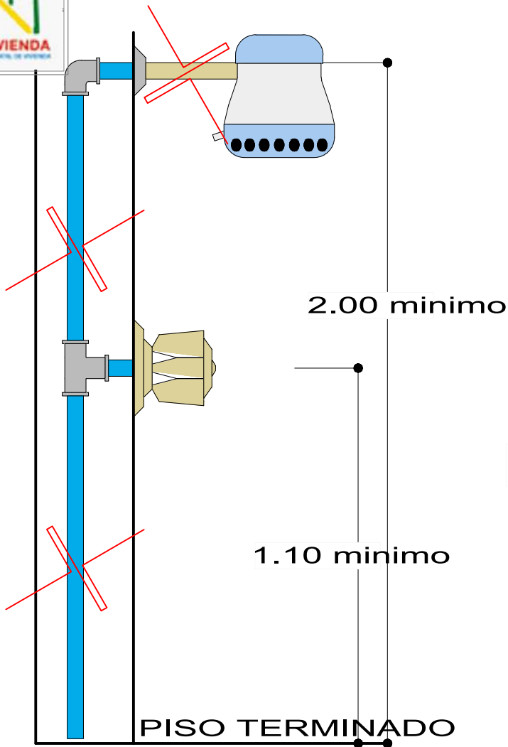
DETALLE DE DUCHA
