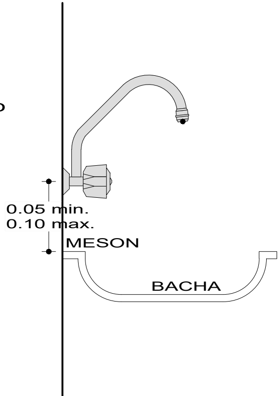
DETALLE DE GRIFO
