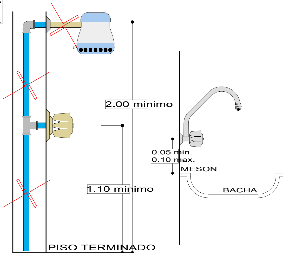
DETALLE DE DUCHA
