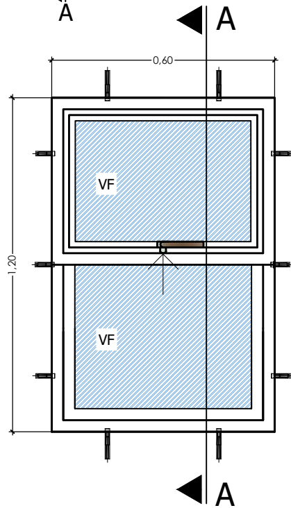
ELEVACION
