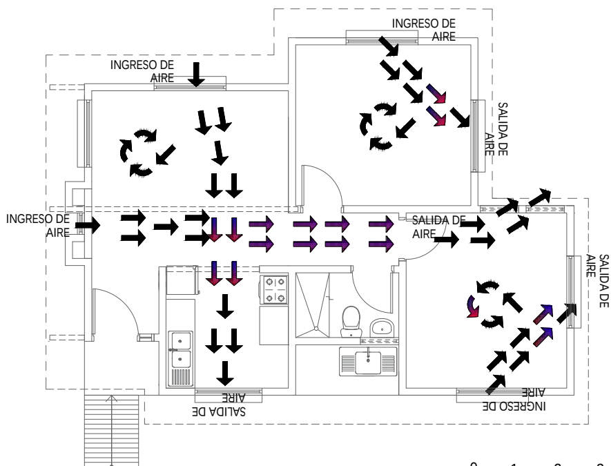
PLANTA CIRCULACION CRUZADA DE AIRE ESC. 1:100
