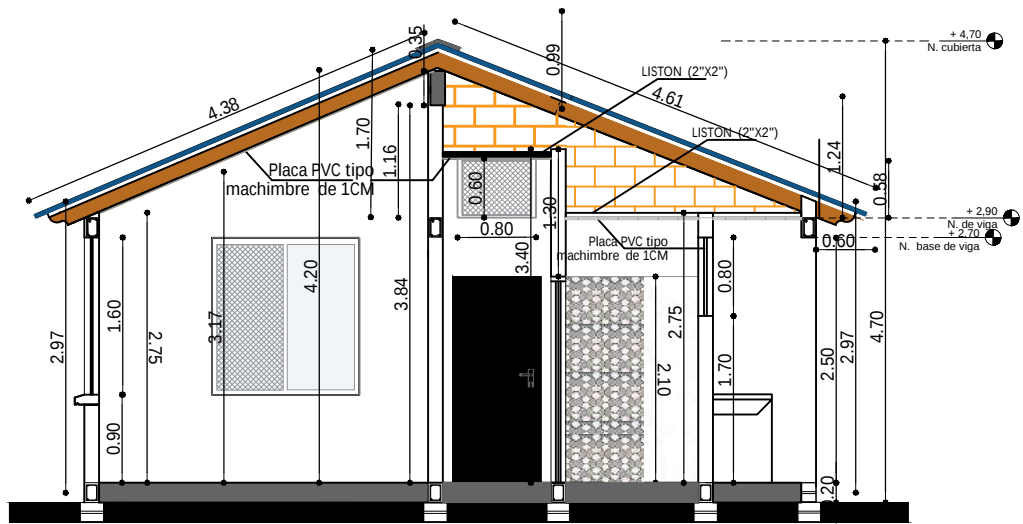
CORTE C-C" ESC. 1:75
