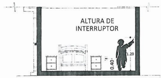
CORTE REFERENCIAL
