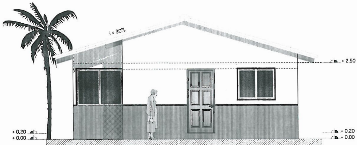
ELEVACIÓN POSTERIOR ESC. 1:75
