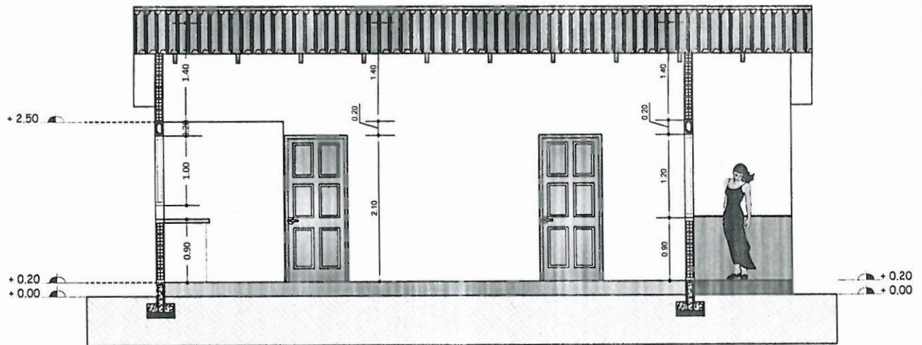
SECCIÓN A-A' ESC. 1:75
