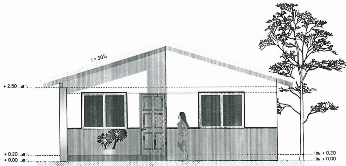
ELEVACIÓN FRONTAL ESC. 1:75
