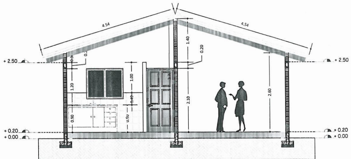
SECCIÓN B-B' ESC. 1:75
