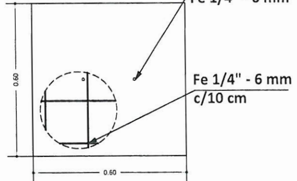
TAPA DE HºAº
