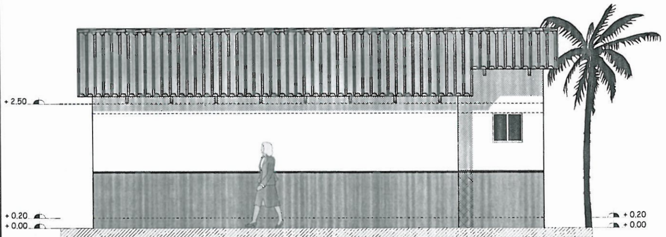
ELEVACIÓN LATERAL DERECHA ESC. 1:75
