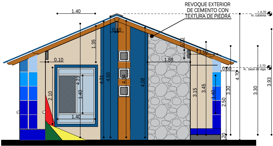
ELEVACION FRONTAL ESC. 1:75
