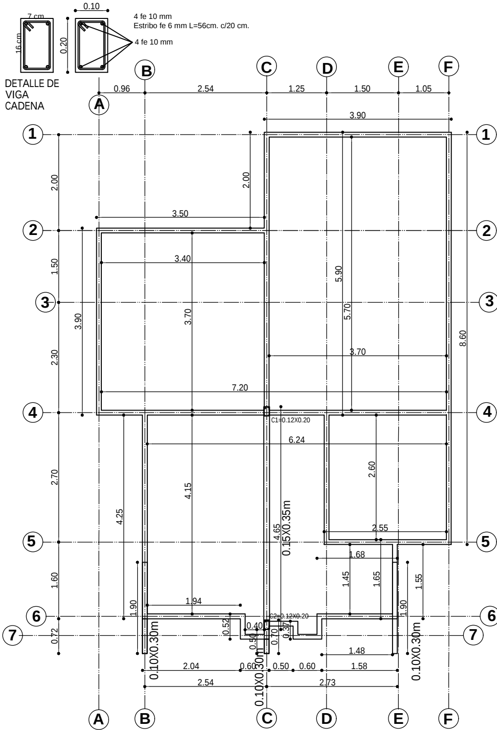
PLANO VIGA CADENA DE H°A° ESC. 1:75
