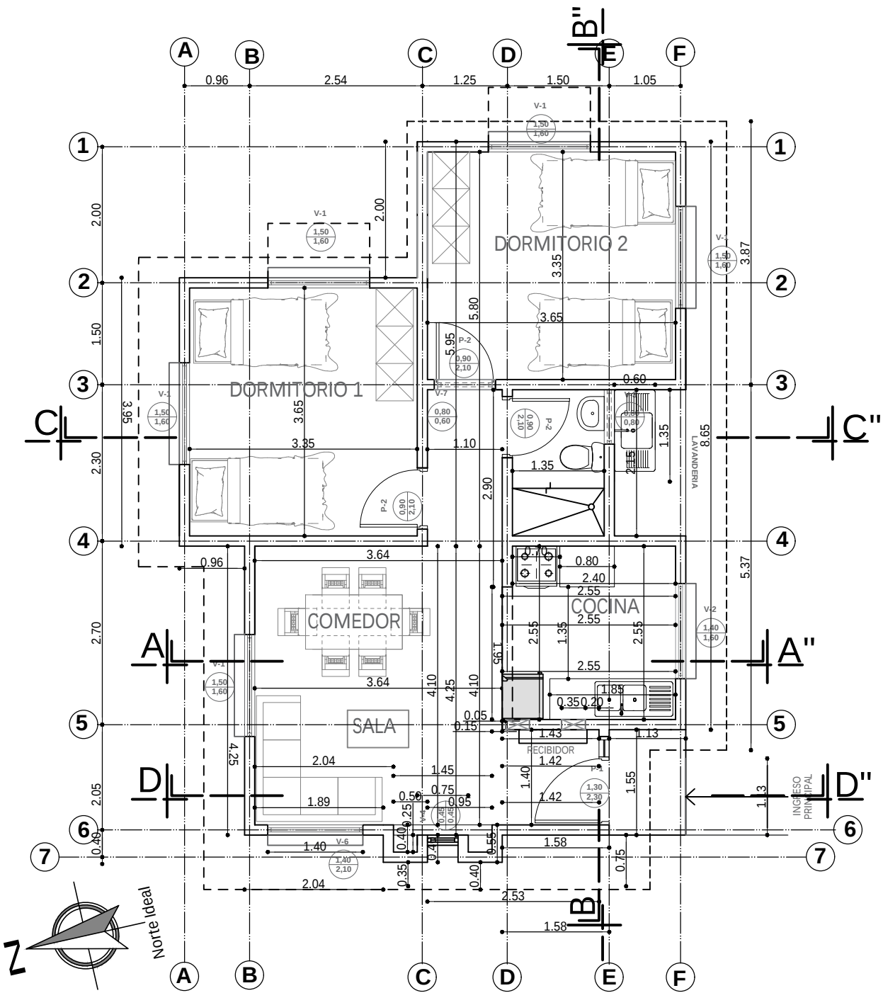
PLANTA ACOTADA ESC. 1:75
