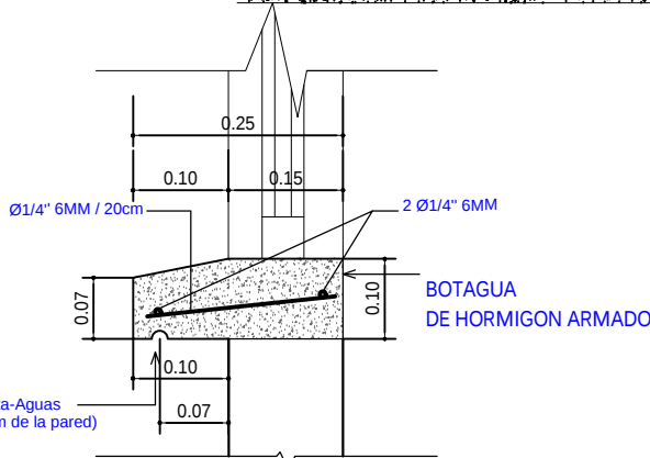
DETALLE DE BOTAGUA ESC. 1:20
